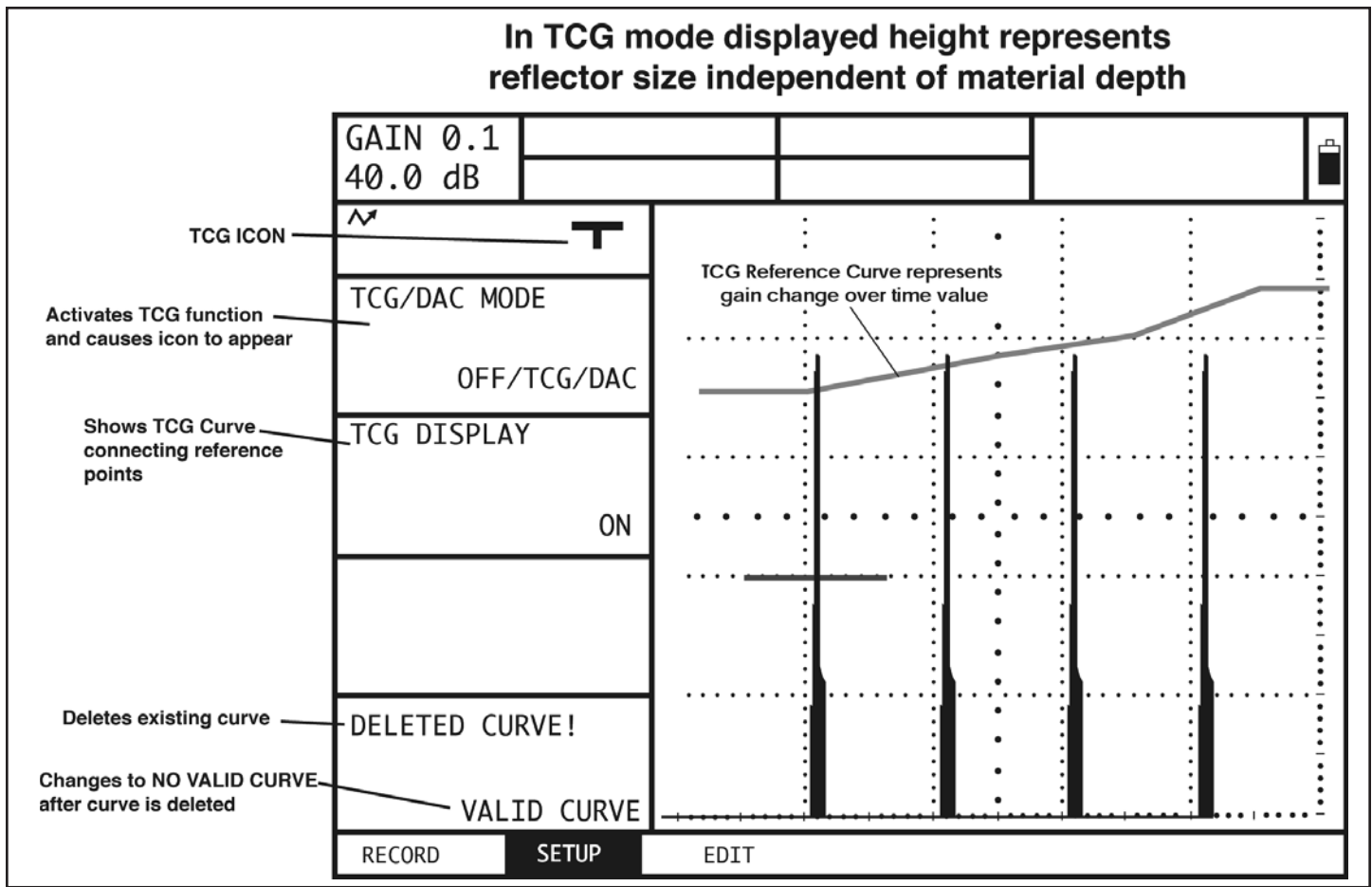
РИСУНОК 5-7—Кривая TCG (ВРЧ)
