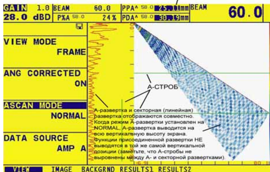
РИСУНОК 3-4—Настройка режима А-развертки привязывает ее вертикальное положение к вертикальному положению соответствующих разверток, или растягивает А-развертку на всю высоту экрана.
