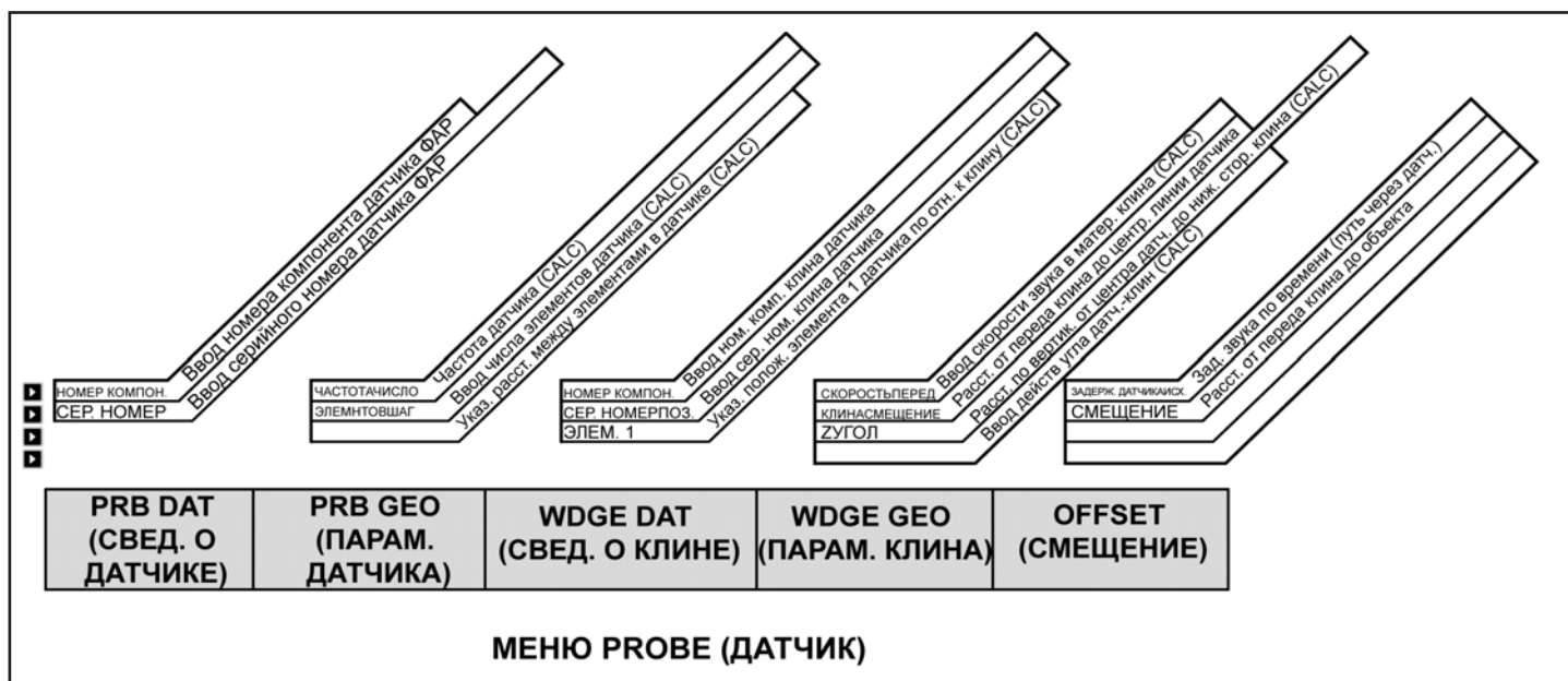
РИСУНОК 2-3— Меню PROBE (ДАТЧИК) позволяет пользователю вводить параметры, связанные с конфигурацией датчика и клина. При изменении значений функций, помеченных CALC, требуется произвести пересчет законов задержки.
