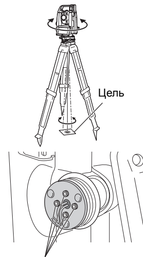
Винты точной регулировки
