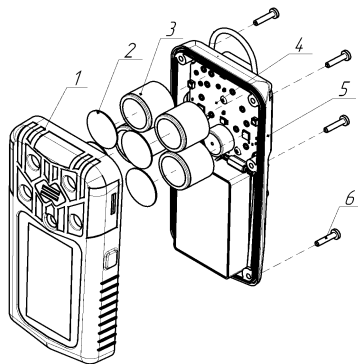
Рисунок 8 – Внешний вид газоанализатора в разобранном состоянии
