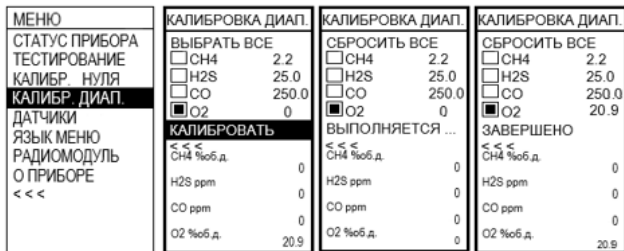
Рисунок 6 – Корректировка диапазона сенсора кислорода
