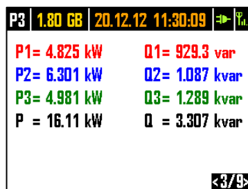
Рис.7. Экран 3/10 с активными и реактивными мощностями.
