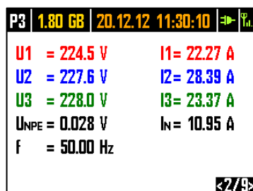
Рис.6. Экран 2/10 с действующими значениями напряжений и токов.
