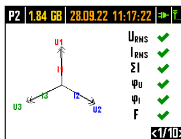
Рис.5. Экран 1/10 с векторной диаграммой.
