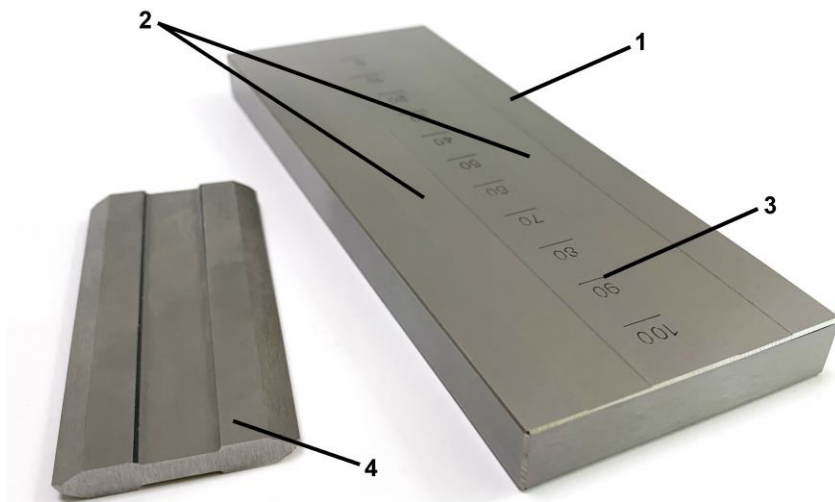
1 – измерительная плита; 2 – паз; 3 – шкала; 4 – скребок.
