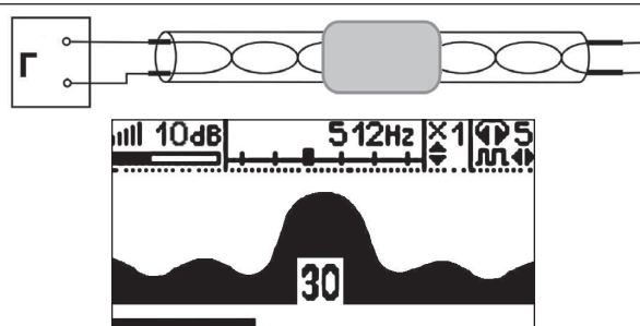
Рис.4.8 Муфта
