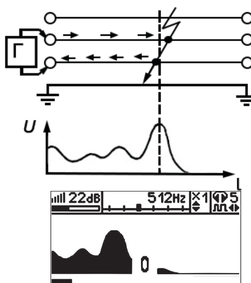
Рис.4.10 КЗ-двухфазное
