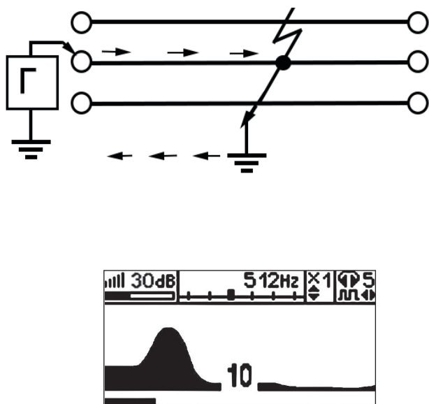
Рис.4.9 КЗ-однофазное
