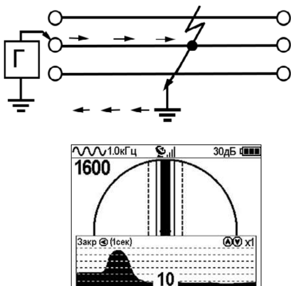
Рис.А.3 КЗ-однофазное
