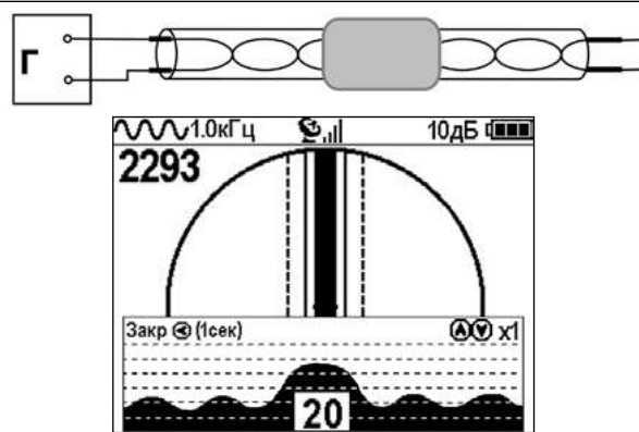
Рис.А.2 Муфта
