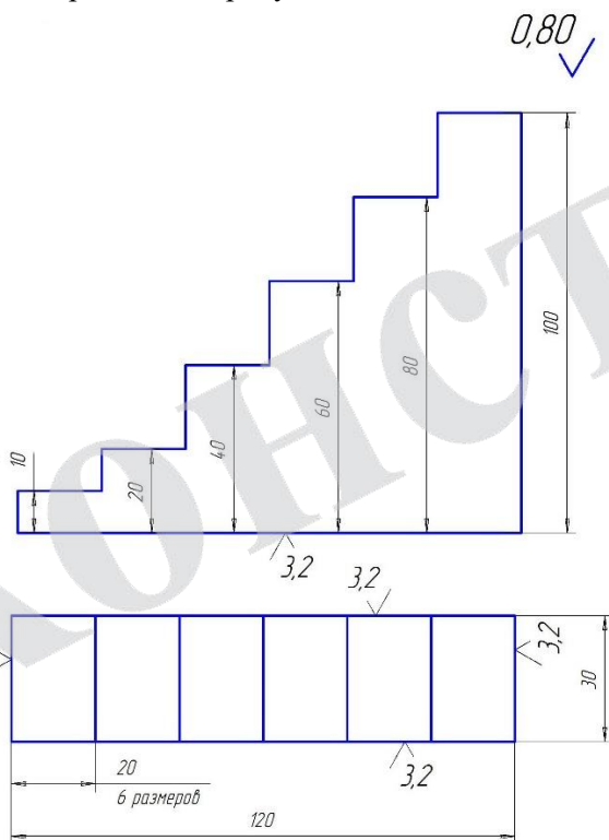
Рисунок 1 – Настроечный образец ОС-3 (эскиз).
