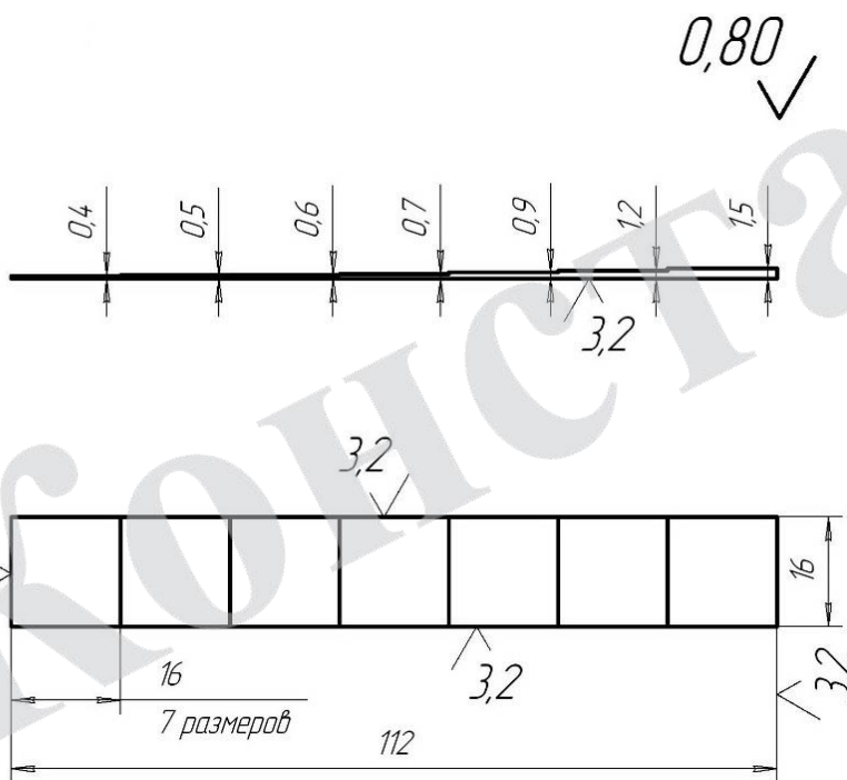
Рисунок 1 – Настроечный образец ОС-19 (эскиз).
