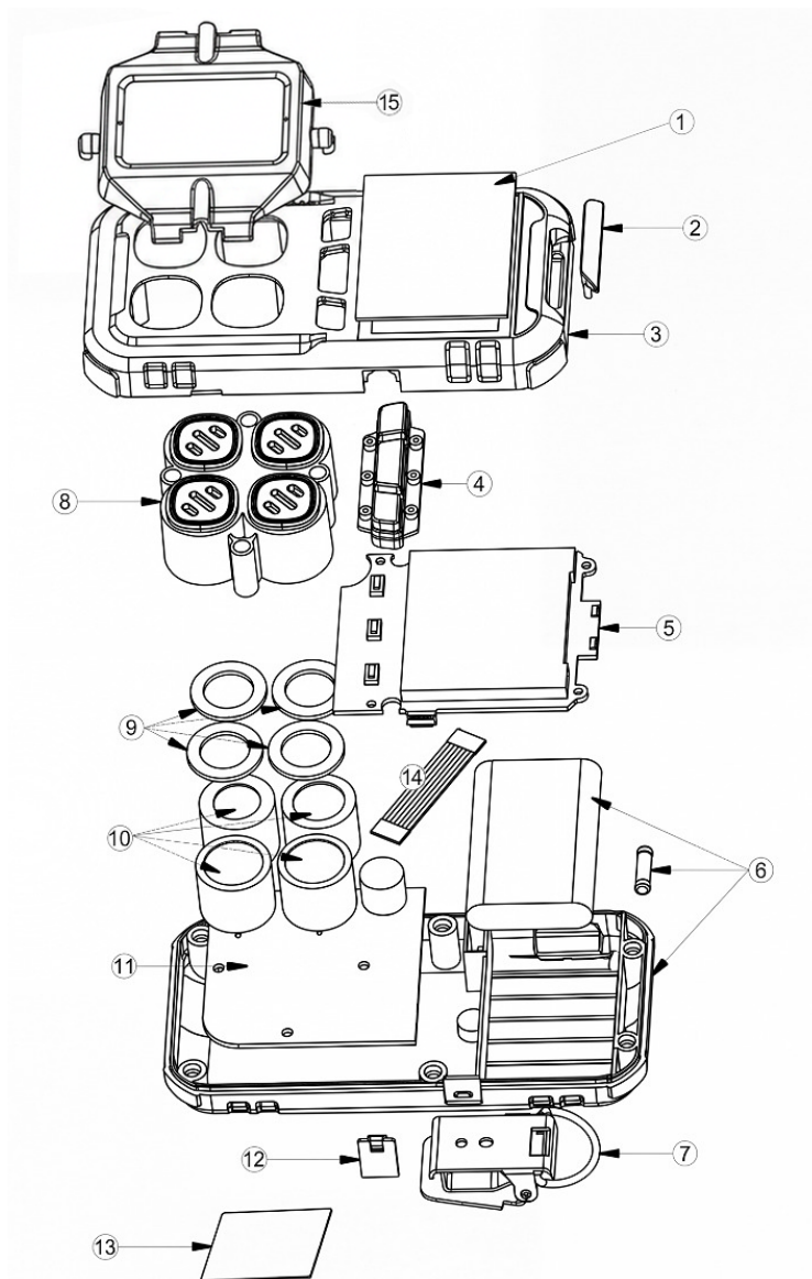
Рисунок 14 - Схема запасных частей
