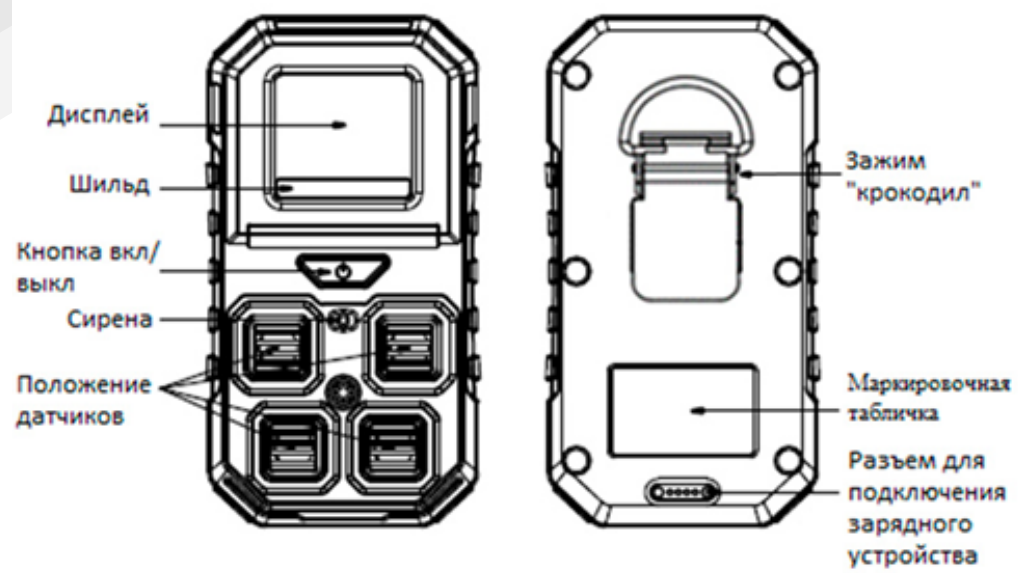
Рисунок 4 - Внешняя конструкция и элементы управления HardGas X4.
