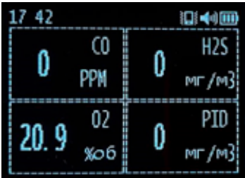
Рисунок 6 – Дисплей HardGas X4 в «основном режиме работы»
