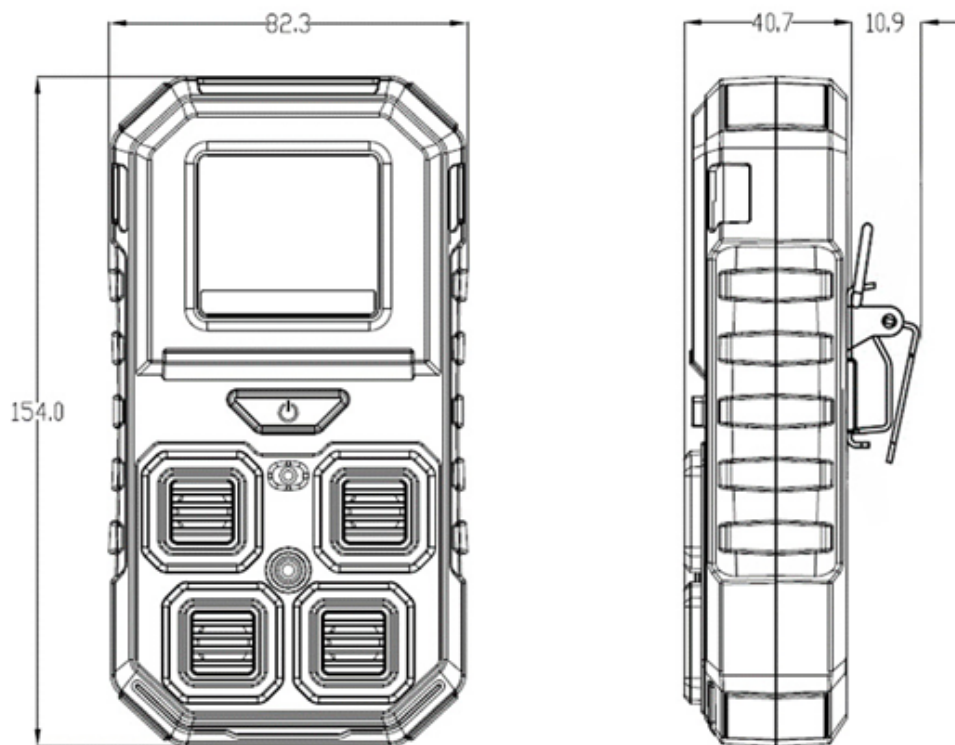
Рисунок 3 – Габаритные размеры HardGas X4.
