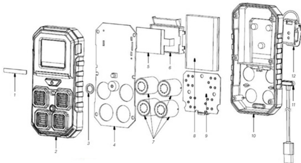
Рисунок 5 – Структурная схема газоанализатора.
