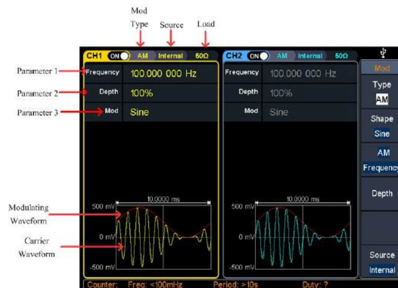
Рисунок 16 - Интерфейс задания настроек модуляции AM
