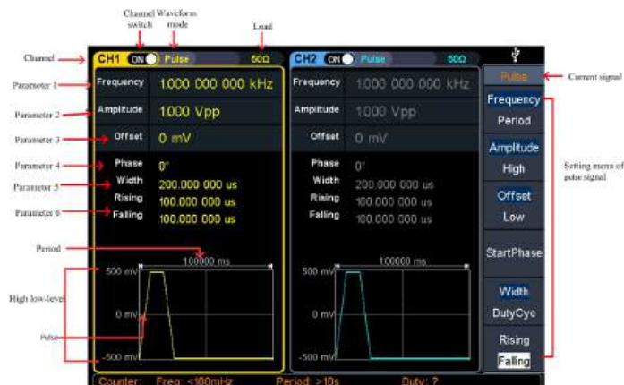
Рисунок 10 - Задание длительности импульса
