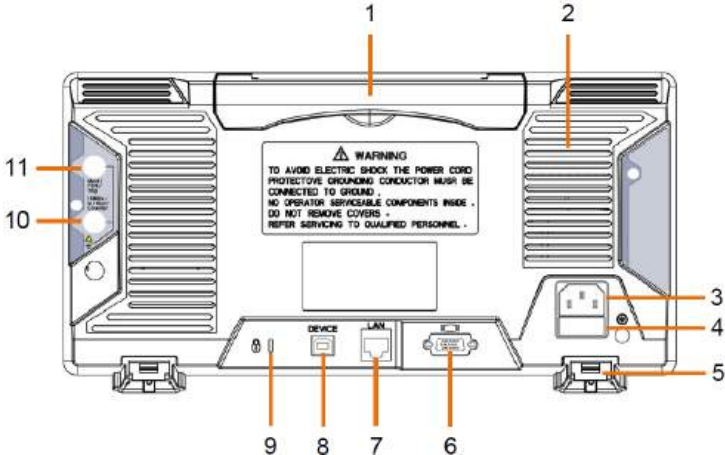
Рисунок 2 - Вид задней панели
