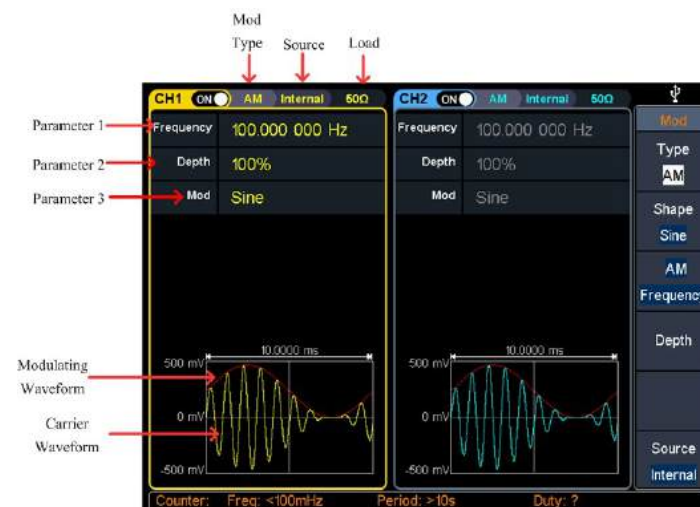
Рисунок 17 - Интерфейс задания параметров DSB-AM
