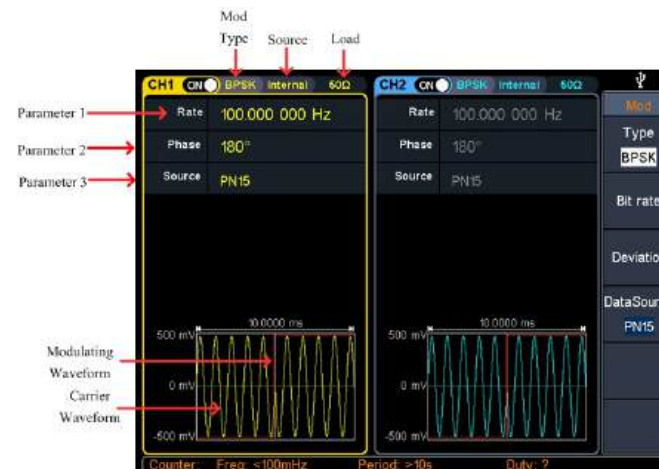
Рисунок 26 - Интерфейс задания настроек BPSK
