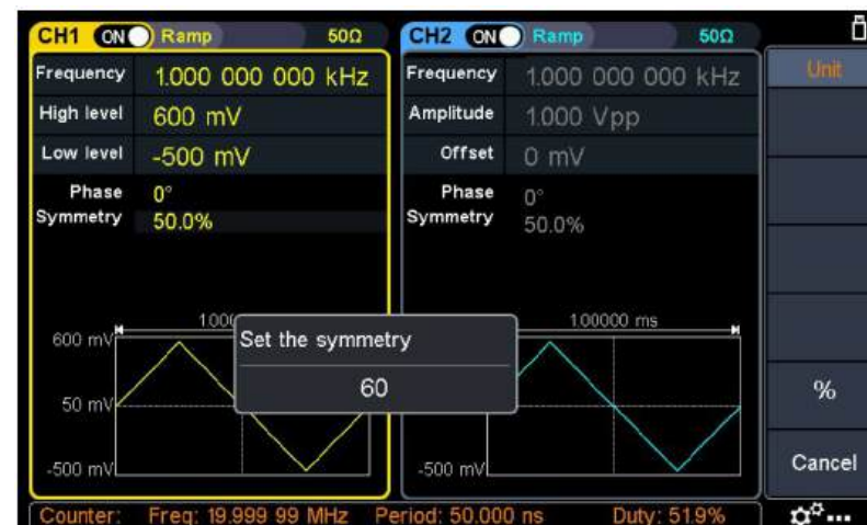
Рисунок 8 - Настройка симметрии пилообразной волны
