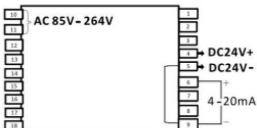
Рисунок 4.2 - Подключение к контроллеру (вариант 1)
