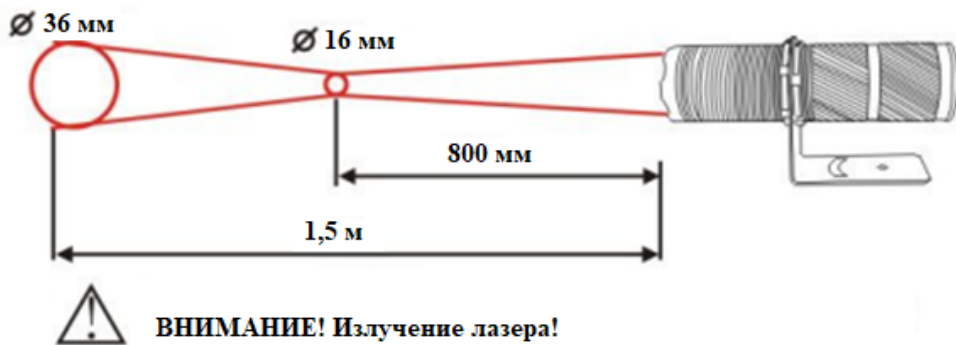
Рисунок 1.1 – Выбор оптимального расстояния для измерения
