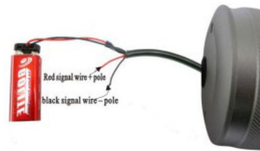
Рисунок 4.1 - Подключение к контроллеру
