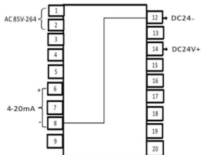
Рисунок 4.3 - Подключение к контроллеру (вариант 2)
