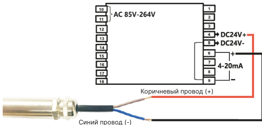
Рисунок 5.1 - Подключение к контроллеру (вариант 1)
