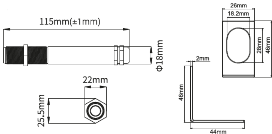
Рисунок 1.1 – габаритный чертёж
