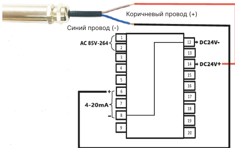
Рисунок 5.2 - Подключение к контроллеру (вариант 2)
