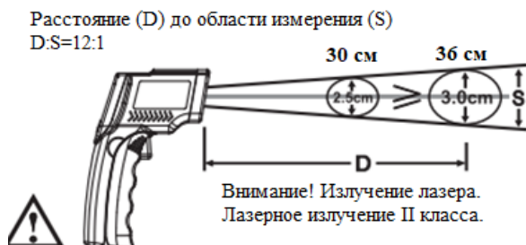
Рисунок 3 - Выбор оптимального расстояния для измерения
