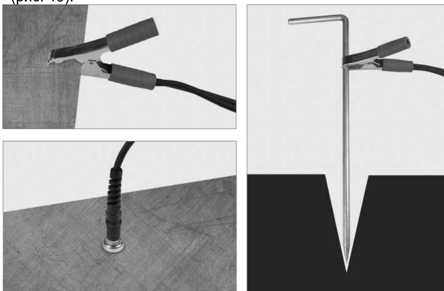
Рис. 19. Подсоединение провода заземления к металлическому изделию с помощью магнита, зажима типа «крокодил» или штыря-заземлителя
