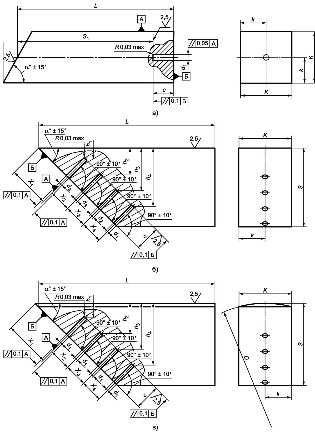
Рисунок 34 — Настроечный образец с плоскдонными отверстиями для ультразвукового контроля наклонными ультразвуковыми преобразователями
