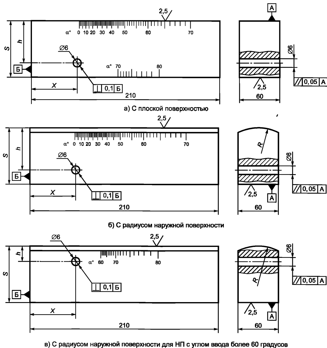
Рисунок 52 — Эскиз НО-СО-2А
