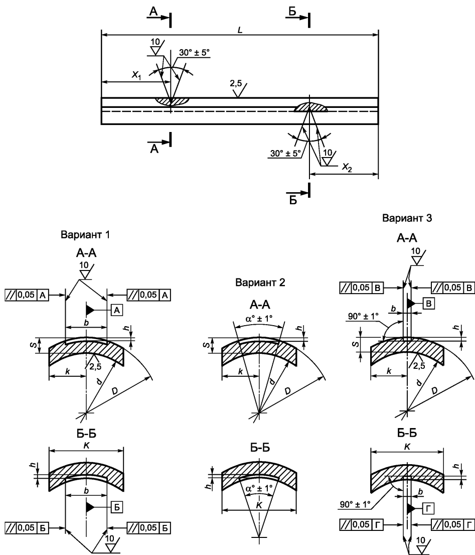
Рисунок 19 — Настроечный образец с рисками
