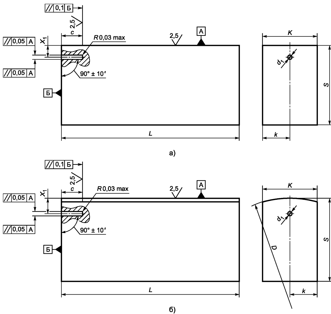
Рисунок 37 — Настроечный образец с плоскостным отверстием для ультразвукового контроля пьезоэлектрическим преобразователем головной волны
