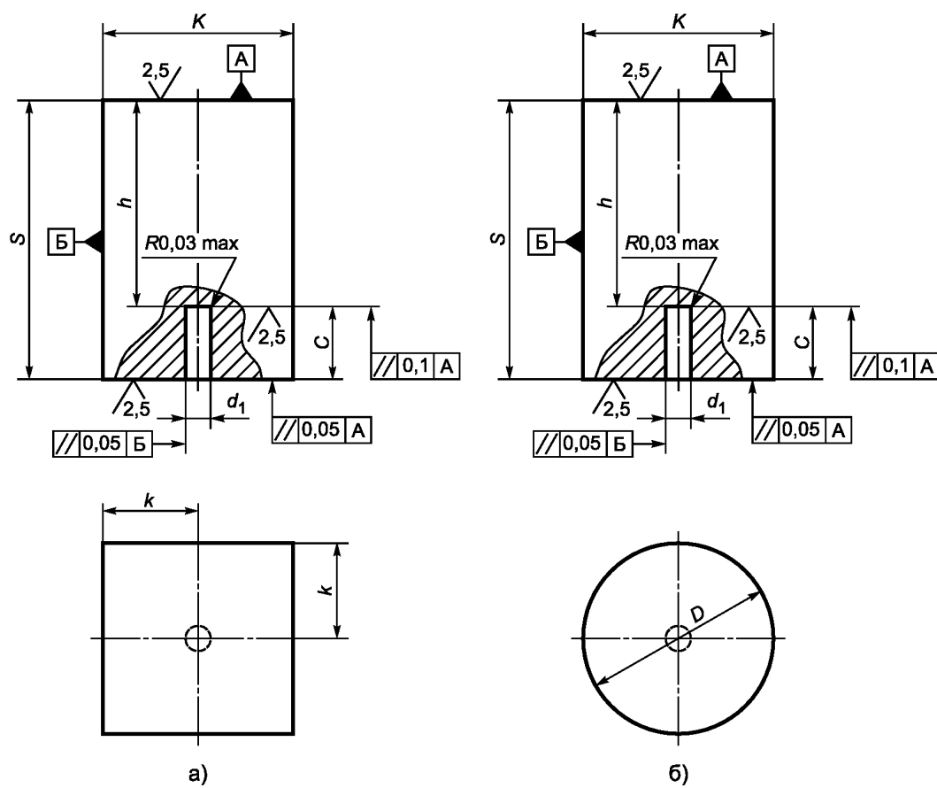
Рисунок 32 — Настроечный образец с плоскодонными отверстиями для ультразвукового контроля прямыми ультразвуковыми преобразователями
