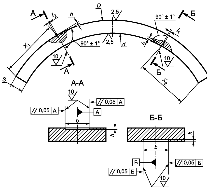
Рисунок 22 — Настроечный образец с непротяженными пазами, выполненными вдоль оси трубы (гиба)
