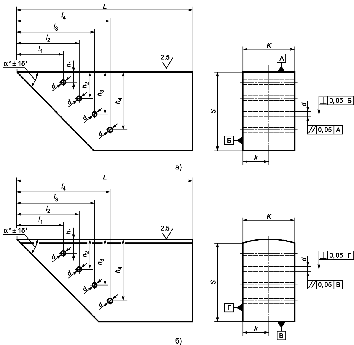
Рисунок 60 — Эскиз настроечного образца для настройки параметров ультразвукового контроля и временной регулировки чувствительности наклонного преобразователя
