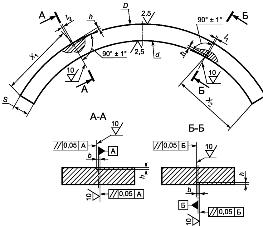
Рисунок 22 — Настроечный образец с непротяженными пазами, выполненными вдоль оси трубы (гиба)
