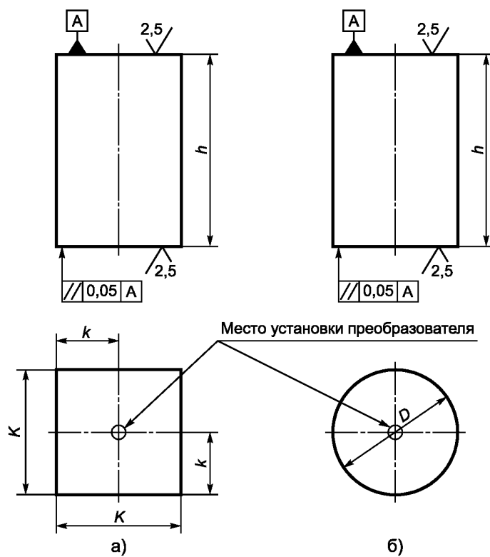
Рисунок 42 — Настроечные образцы для измерения толщины монометаллов (тип Т2)
