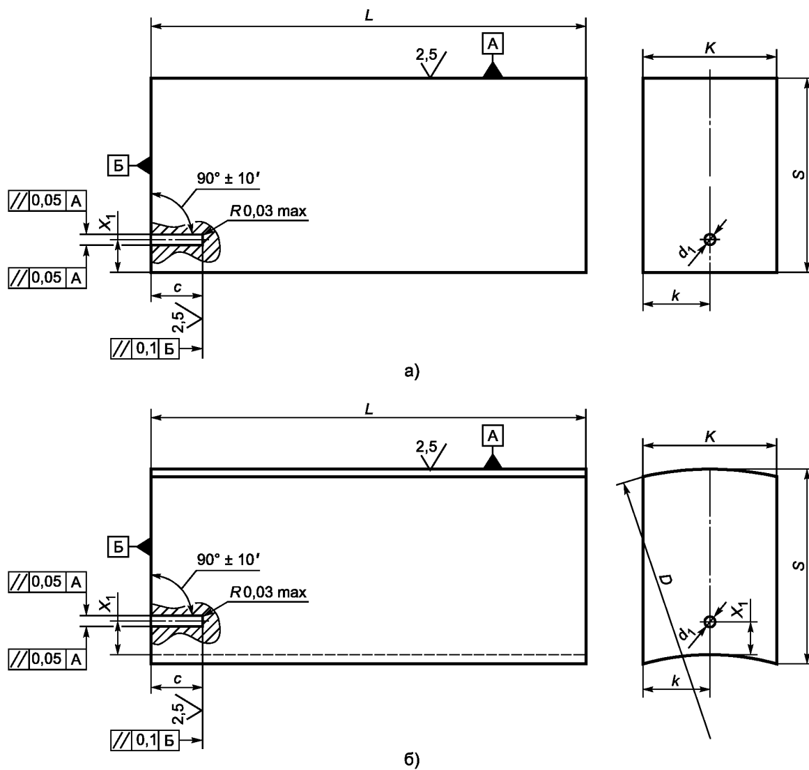
Рисунок 38 — Настроечный образец с плоскдонным отверстием для ультразвукового контроля пьезоэлектрическим преобразователем «корневой тандем»
