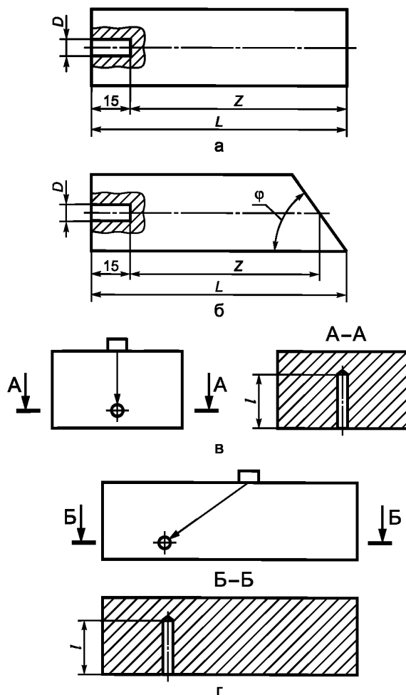
Рисунок 5 — Настроечные образцы
