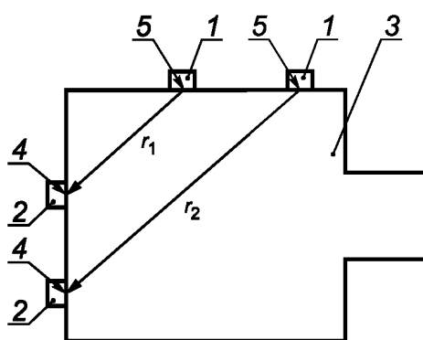
1 — излучатель; 2 — приемник; 3 — ОК; 4, 5 — точки ввода
