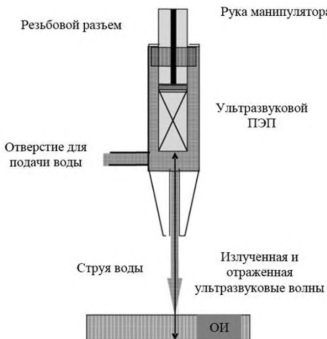
Рисунок 1 — Метод А. Автоматизированный ультразвуковой эхо-импульсный метод
