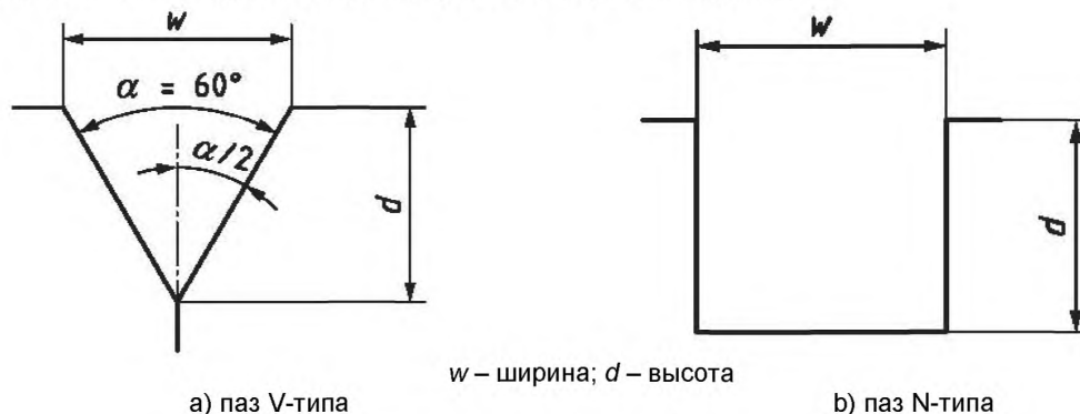
Рисунок 1 – Типы пазов
