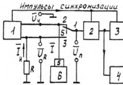
1 — генератор импульсов возбуждения; 2 — приемник; 3 — осциллограф; 4 — анализатор спектра; 5 — проверяемый ПЭП; 6 — акустическая нагрузка
