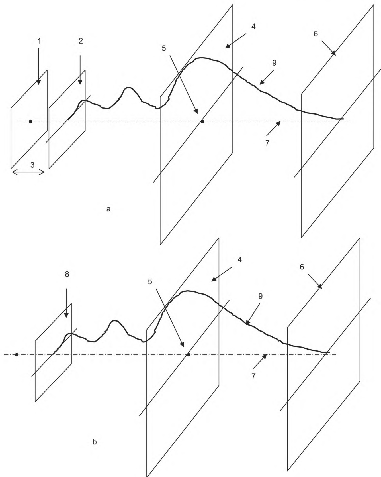
Рисунок 9 — Фокус в поле давлений на главной продольной плоскости для преобразователя известной (а) и неизвестной (б) конструкции
