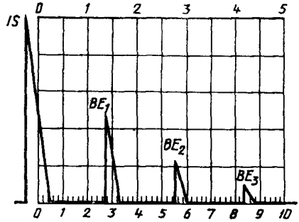
Удовлетворительное соединение
