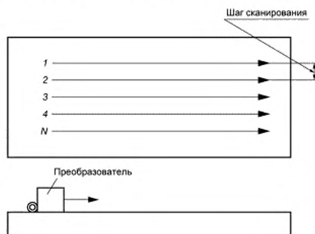
Рисунок 9 — УЗКТ непрерывным сканированием участка поверхности
