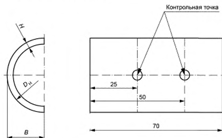
Рисунок 17 — Настроечный образец в виде участка трубы
