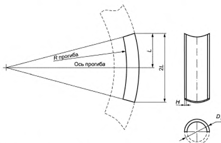
Рисунок 18 — Настроечный образец в виде участкагиба (колена) трубопровода
