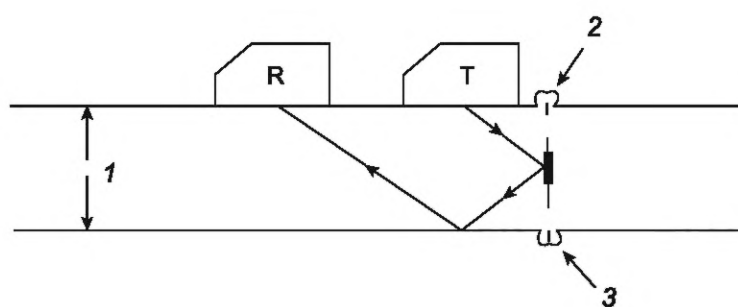
Рисунок 5 — Контроль методом тандем
