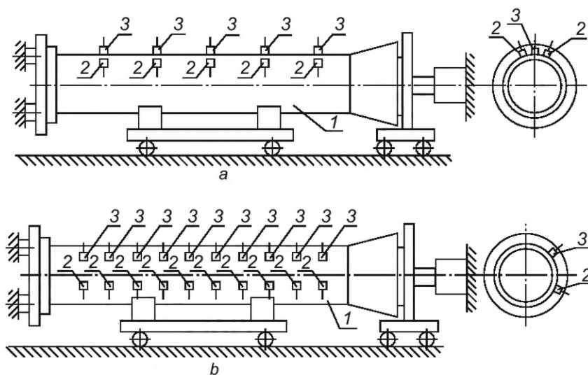
1 — труба; 2 — излучатели; 3 — приемники
