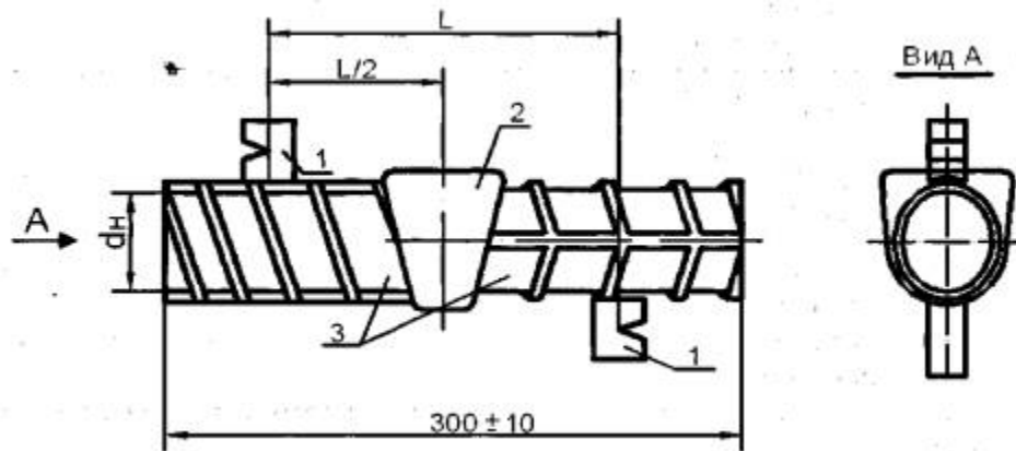
Рис. 1. Схема ультразвукового контроля сварного стыкового соединения арматурных стержней теньвым методом.
