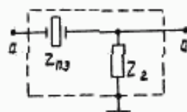
Z_{\text{н.з}} — проверяемый ПЭП; Z_2 — электрическая нагрузка
