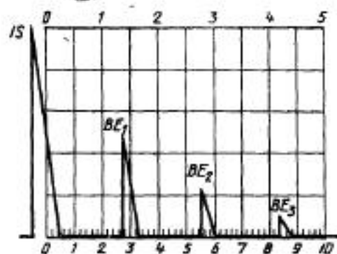
Удовлетворительное соединение
