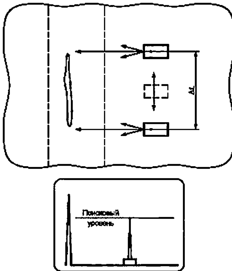
Рисунок В.7 — Схема измерения условной протяженности дефекта
