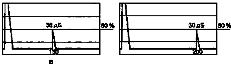
Рисунок Ж.1 — Экран дефектоскопа при измерении амплитуды эхо-сигнала
