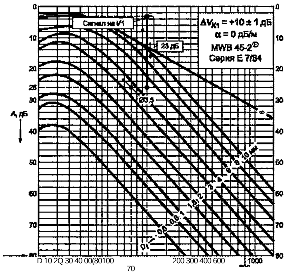
Рисунок Ж.8 — Определение эквивалентной площади по АРД-диаграммам с использованием образца Y1
