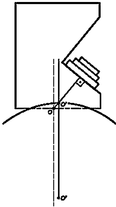
О и О' — точки выхода луча ПЭП с плоской контактной (до проточки) и обработанной поверхностями
