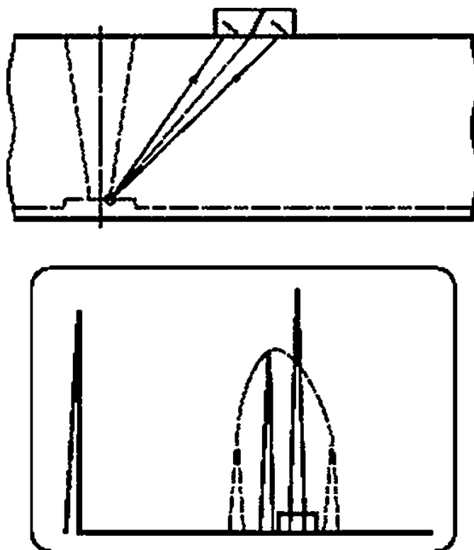
Рисунок В.6 — Схема обнаружения и интерпретации объемных несплошностей под «плавленным покрытием»
