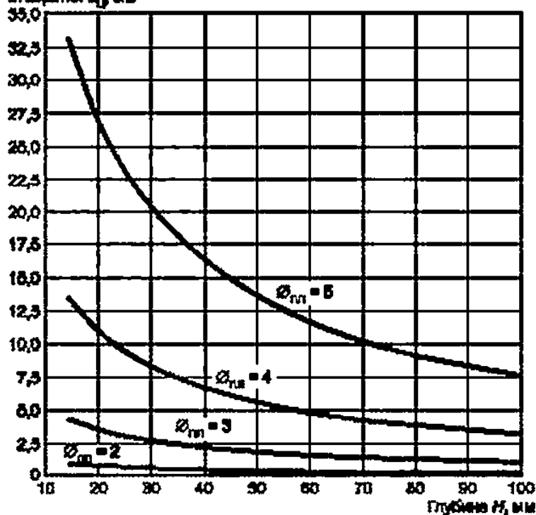
Рисунок Ж.19 — Соотношения между диаметрами бокового цилиндрического и плоскостного отверстий при различной глубине залегания для ПЭП WB 45-2
