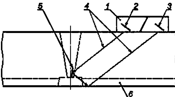
Т — ПЭП. 2, 3 — излучающий и приемный элементы. 4 — направление кода УЗ-колебаний. 5 — трещина под наплавленным покрытием, 6 — антикоррозионное покрытие
