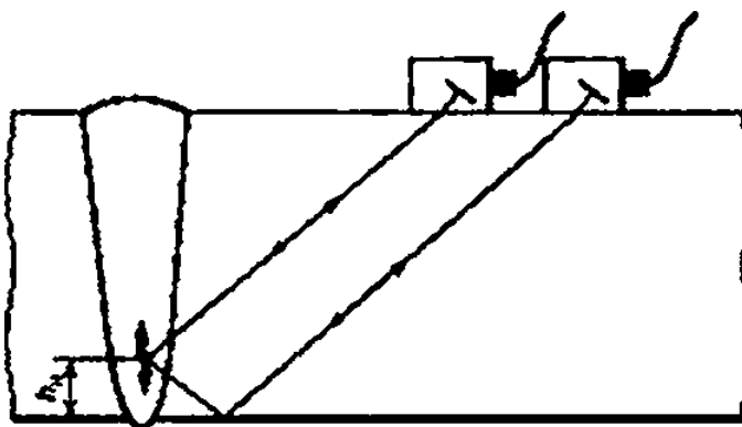
Рисунок К.2 — Зона непрозвучивания h_{\text{М}} при измерении коэффициента формы неслошности
