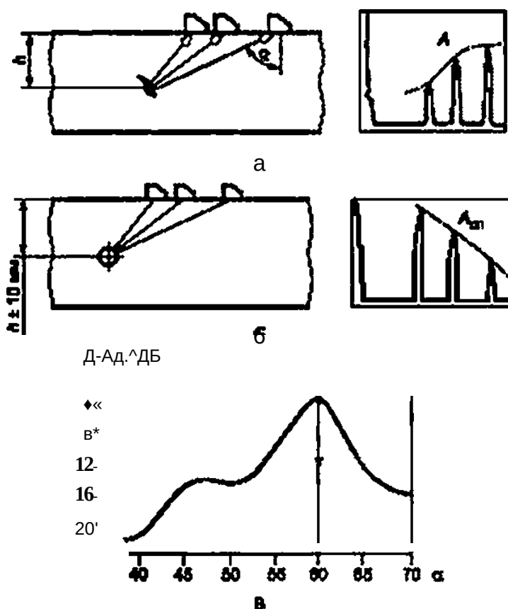
Рисунок Л.1 — Схемы определения ориентации несплошности
