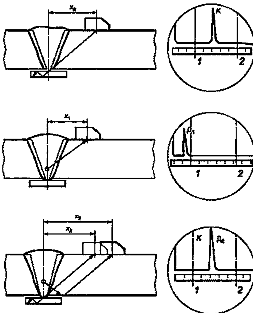
Т и 2 — положение сигналов от углового отражателя; К — сигнал от подкладного кольца. Д 1 и Д 2 — сигналы от надкорневой несплошности, обнаруженные прямым или однократно отраженным лучом: x_k , ж, и *j — расстояния между серединой шва и точкой ввода ПЭП
