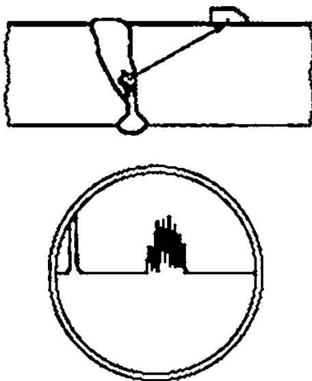
Рисунок М.9 — Выявление рыхлости в СС сосудов
