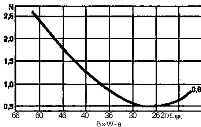
Рисунок Ж.21 — Зависимость N = f(\gamma) для стали, алюминия и его сплавов, титана и его сплавов
