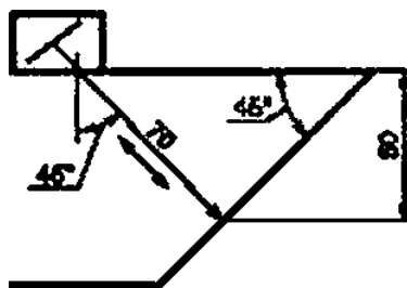
Рисунок Ж.5 — Получение донного сигнала на НО
