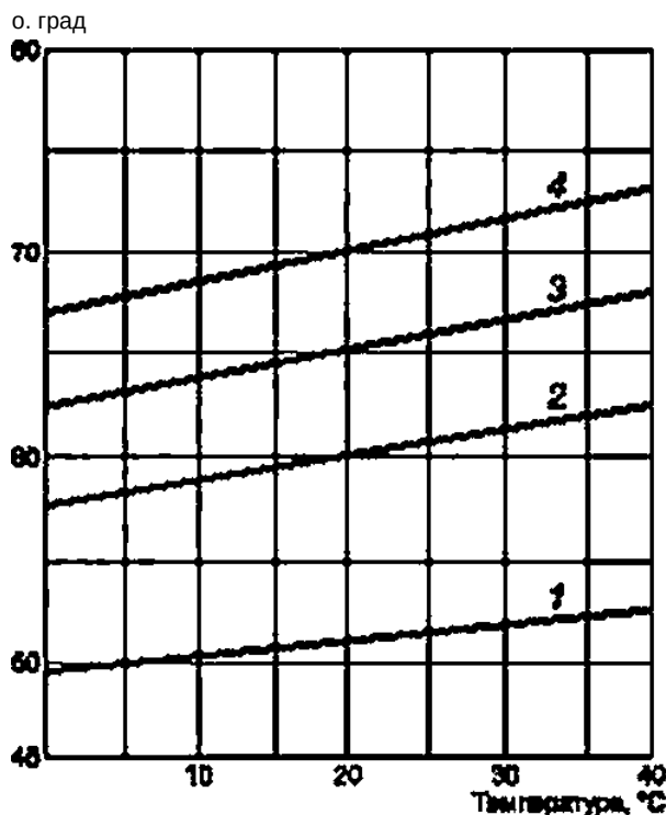
Рисунок 11 — Зависимость угла ввода (α) от температуры для ПЭП с номинальными углами ввода « * 51° (ρ * 40°) (1); 60° (2); 65° (ρ = 50°) (3) и 70° (4)
