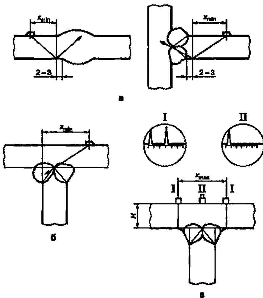
Рисунок М.11 — Определение границ зон перемещения ПЭГП при УЗК СС листовых конструкций
