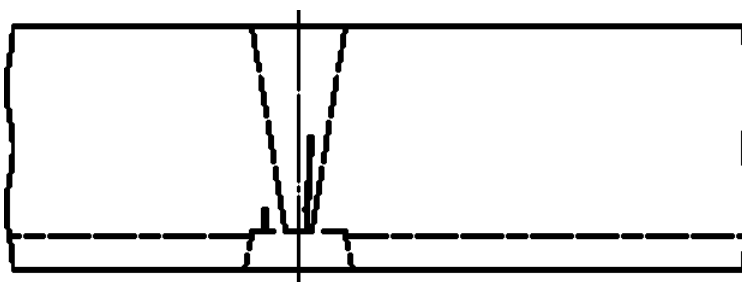
Рисунок В.1 — Трещины под наплавленным аустенитным покрытием на сварное соединение
