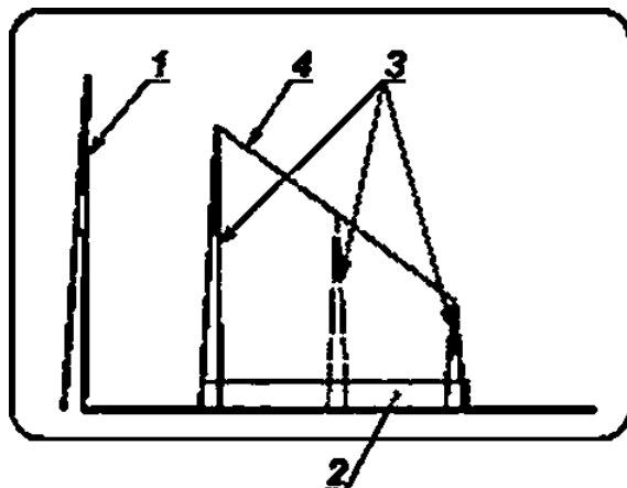
1 — зондирующий импульс, 2 — зона контроля (строб-импульс). 3 — импульсы, отраженные от плоскостонного отверстия в НО. 4 — уровень чувствительности УЗК
