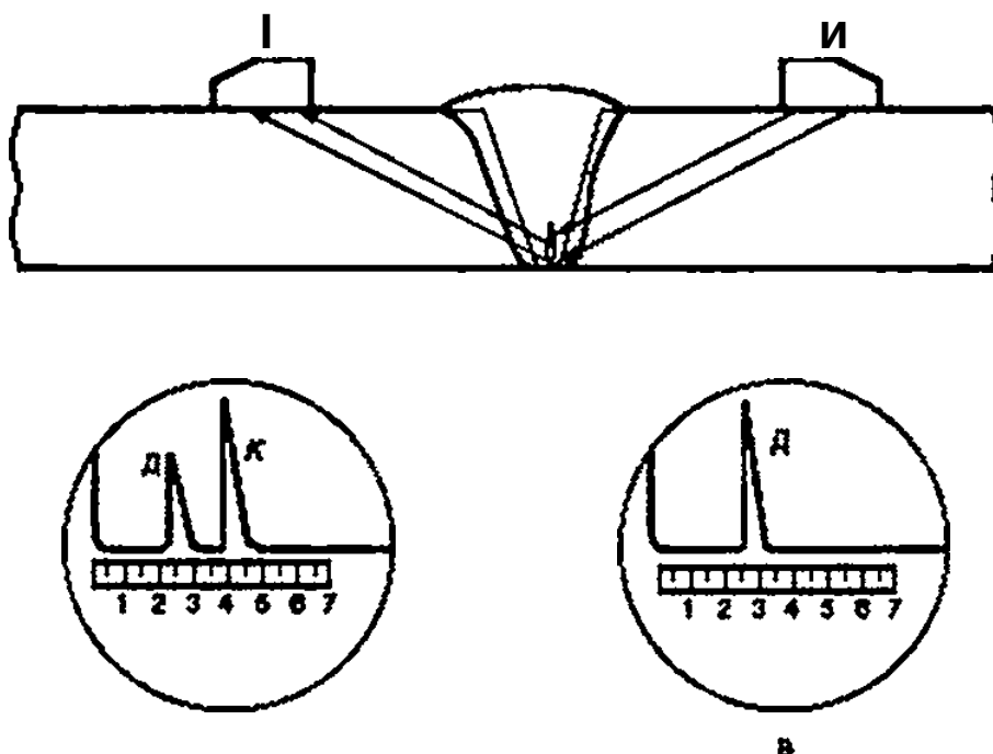
а — схема обнаружения трещины; б — осциллограмма при положении ПЭП I; в — осциллограмма при положении ПЭП II: Д — сигнал от неслошности; К — сигнал от подкладного кольца
