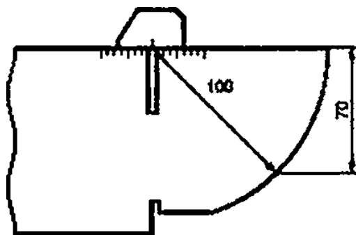
Рисунок Ж. 10 — Получение максимального сигнала на образце VI
