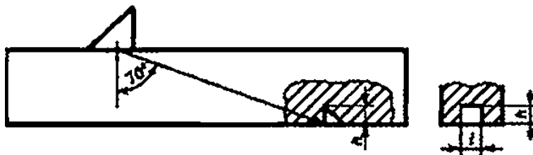
Рисунок Ж.20 — Настройка на ФН с зарубкой
