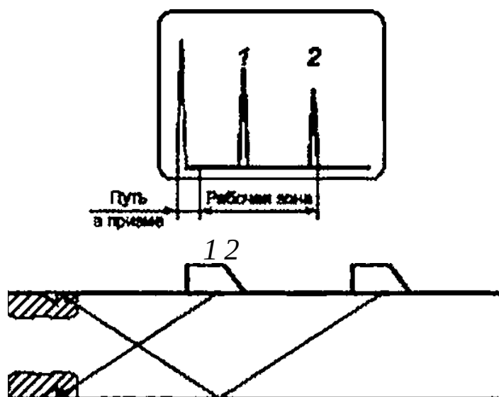
Рисунок 7 — Схема настройки развертки по угловым отражателям
