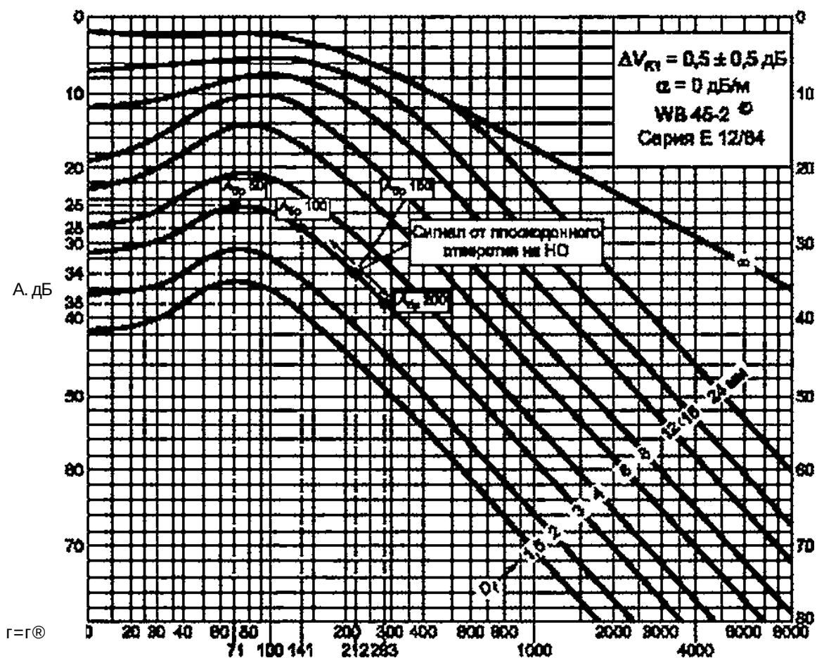
Рисунок Ж.13 — Настройка чувствительности дефектоскопа с использованием АРД-диаграммы и НО с плоскородными отверстиями
