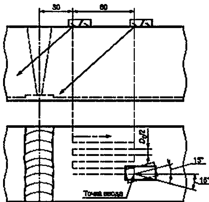
Рисунок В.5 — Схема сканирования
