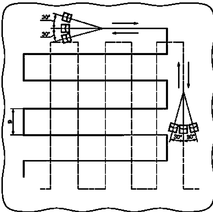
Рисунок Е.3 — Траектория сканирования поверхности наплавленного покрытия (стрелками показаны направления перемещения ПЭГ)
