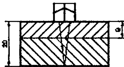
Рисунок Ж.17— НО для УЗК Антикоррозионной наплавки
