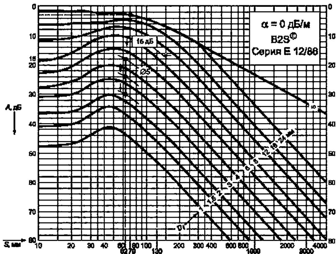
Рисунок Ж.4 — Определение браковочного, контрольного и поискового уровней при УЗК антикоррозионной наплавки
