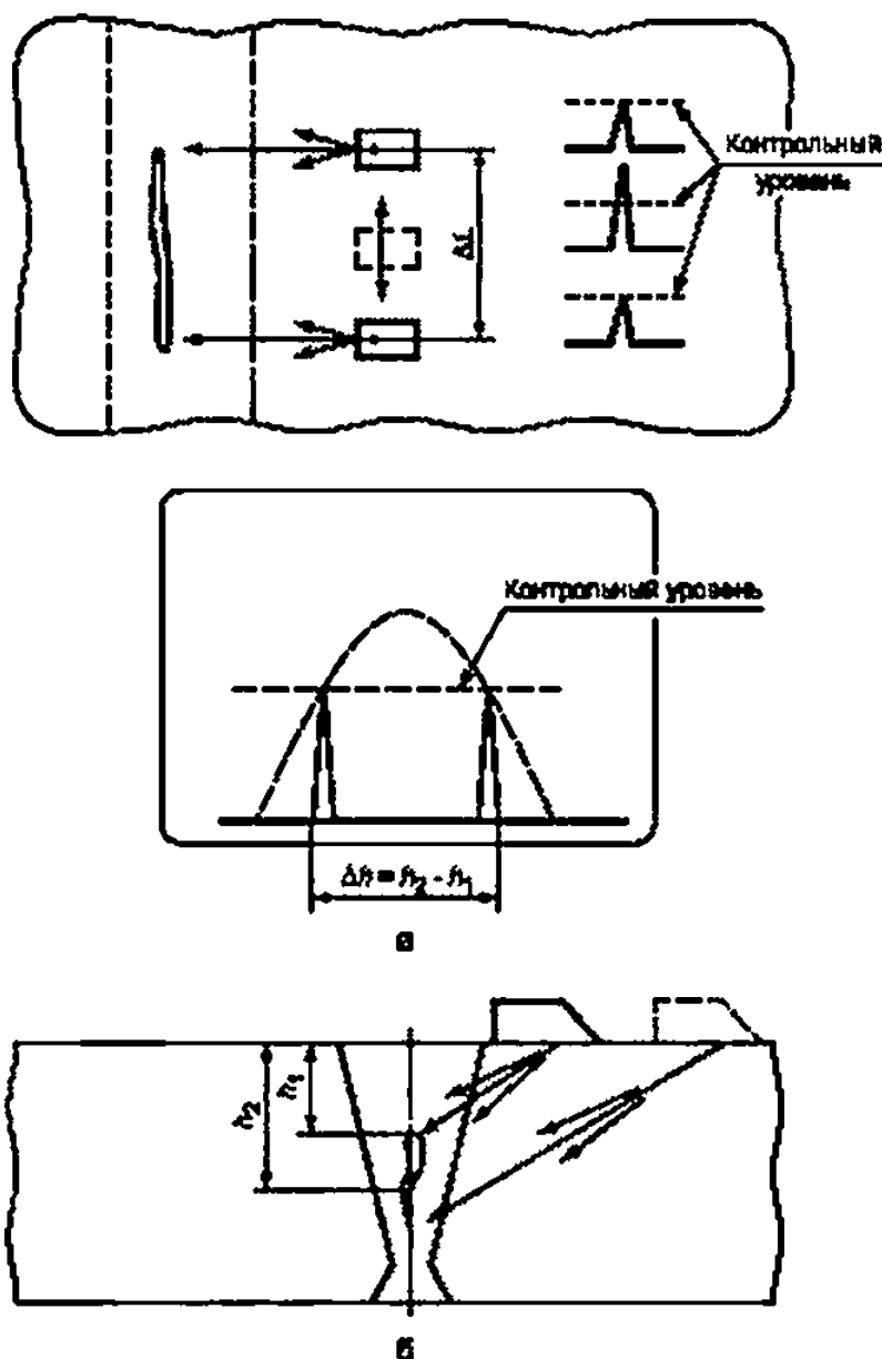
Рисунок 16 — Схемы измерения условной протяженности (а) и условной высоты (б) несплошности
