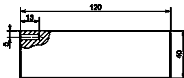
Рисунок Г.2 — Настройочный образец
