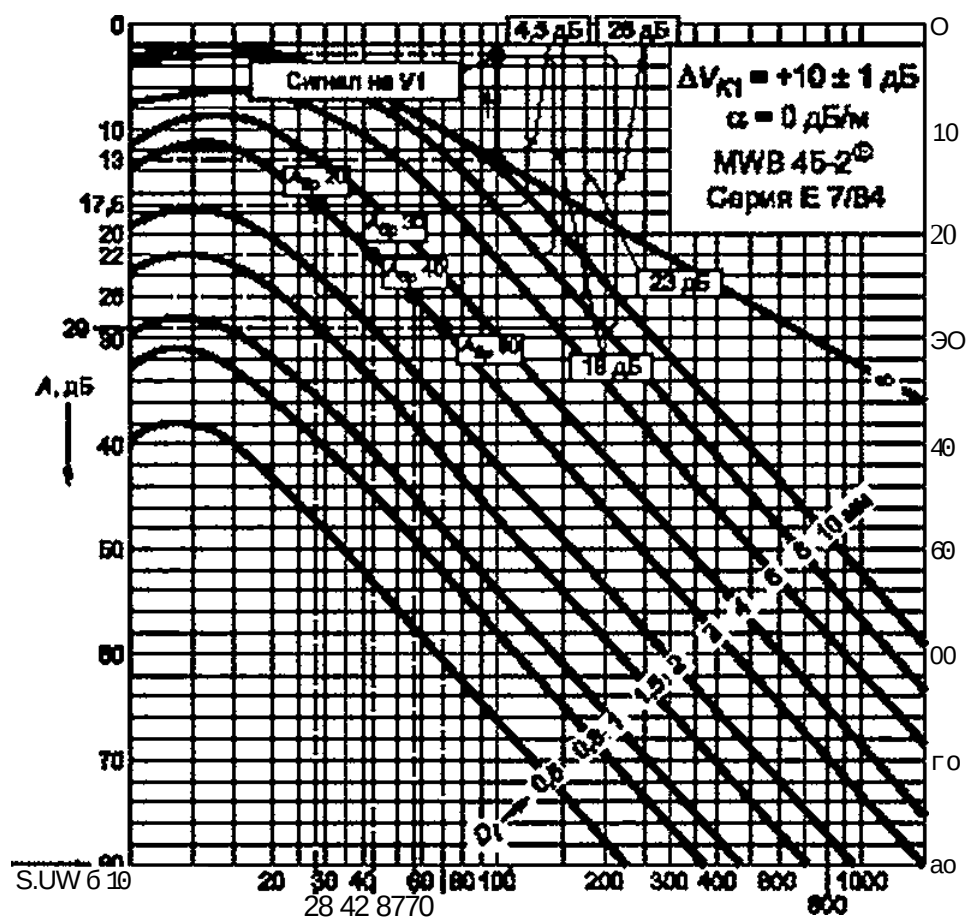
Рисунок Ж.11 — Настройка чувствительности дефектоскопа с использованием АРД-диаграммы и КО У1
