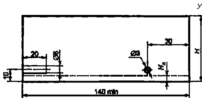
Рисунок В.3 — Настроечный образец ИО-КТ-Ду850
