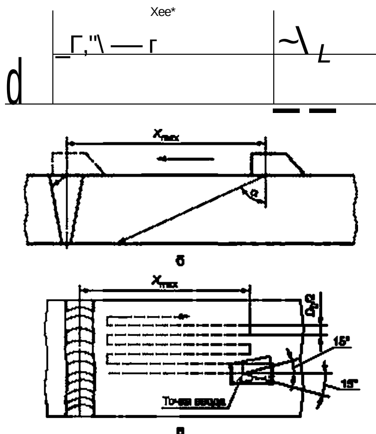
а — при УЗК СС толщиной менее 60 мм; б — при УЗК СС толщиной 60 мм и более; е — траектория сканирования: X до — максимальное удаление ПЭП от шва
