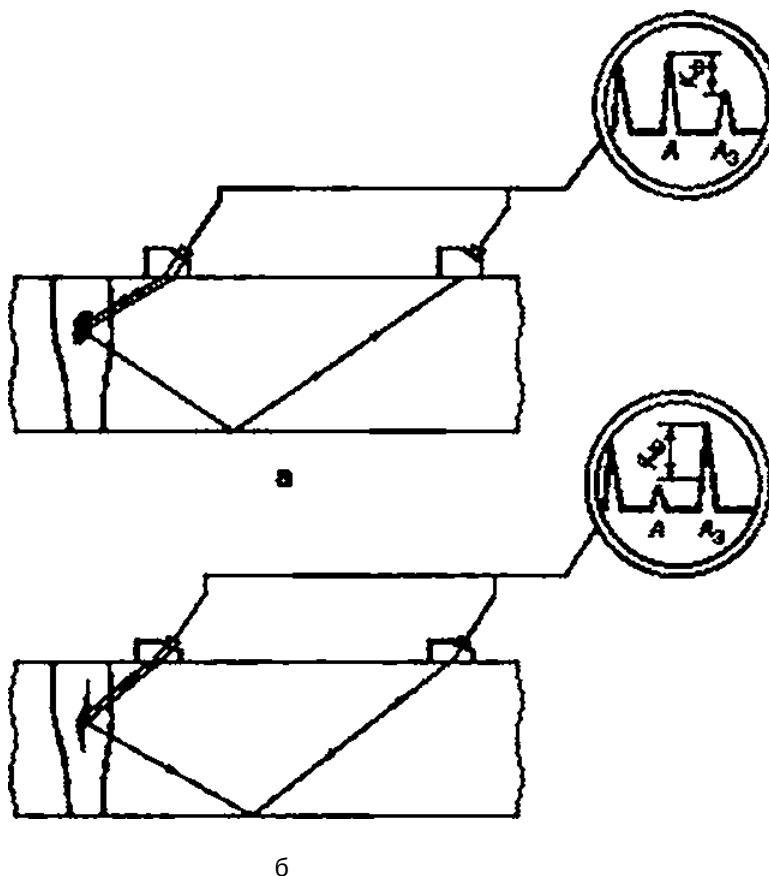
Рисунок К.1—Коэффициент формы плоскостных (а) и объемных (б) несплошностей
