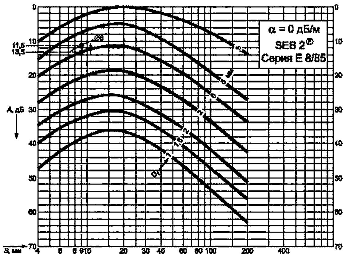
Рисунок Ж.15 — НО для УЗК антикоррозионного наплавленного покрытия с плоскостонным отверстием
