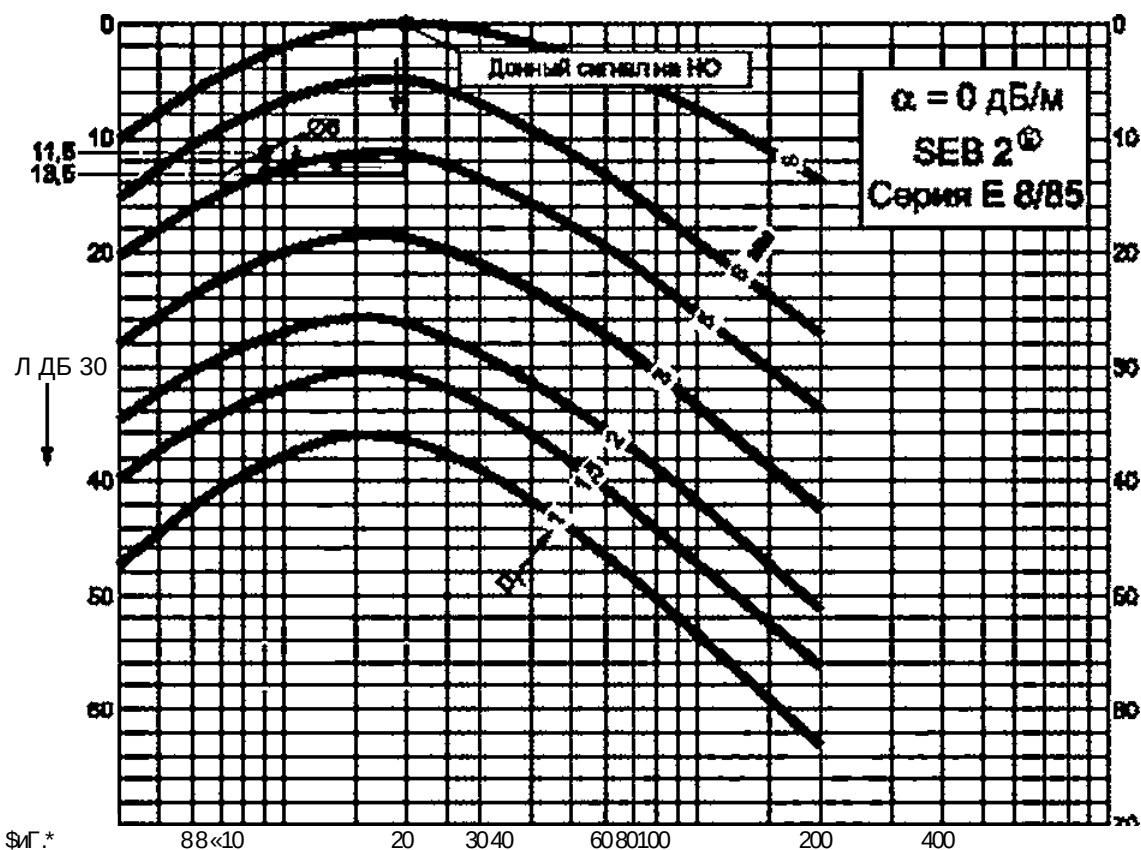
Рисунок Ж.18—Настройка чувствительности и градуировка вальной площади наплавки по АРД-диаграммам с использованием НО
