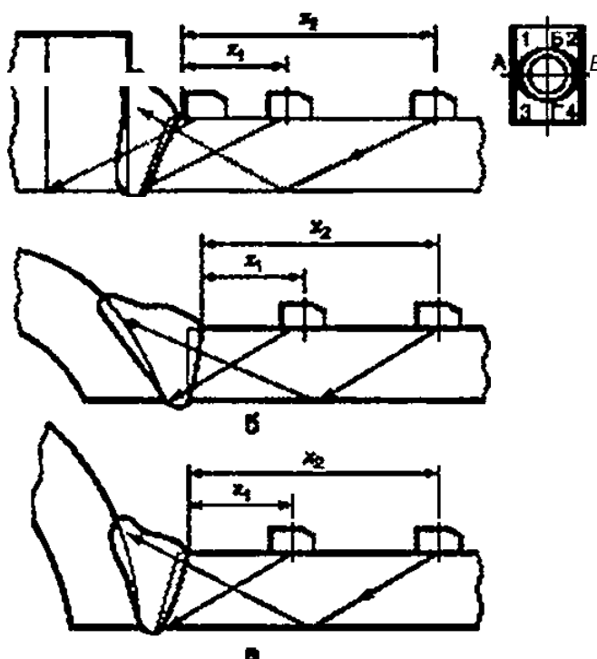
Рисунок М.6 — Схемы УЗК углового кольцевого сварного соединения
