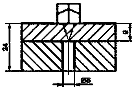
Рисунок Ж.15 — НО для УЗК антикоррозионного наплавленного покрытия с плоскостонным отверстием
