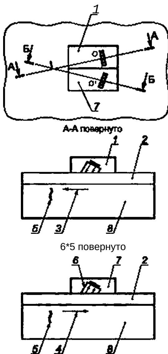
1 — излучатель; 2 — наплавленное покрытие; 3, 4 — продольно-поперечные волны; 5 — трещина; 6 — боковая волна; 7 — приемник; 8 — основной металл
