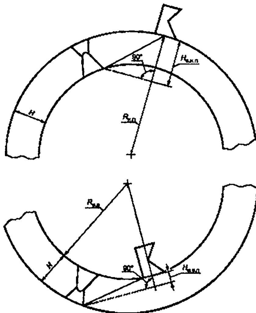
Рисунок Б.1 — Эквивалентная толщина M_{\text{пл}} H_{\text{экв.п}} плоского СС изделий цилиндрической формы
