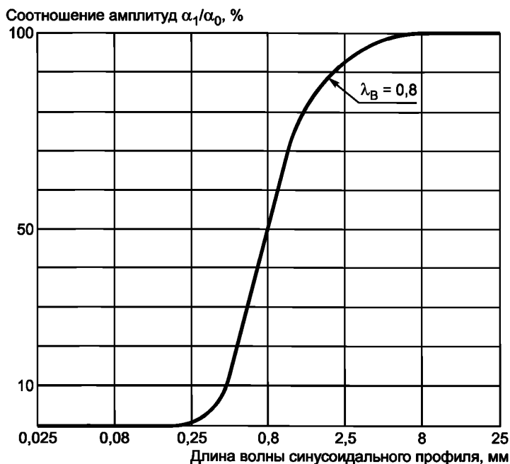
Рисунок 2 — Передаточная характеристика длинноволновой составляющей профиля
