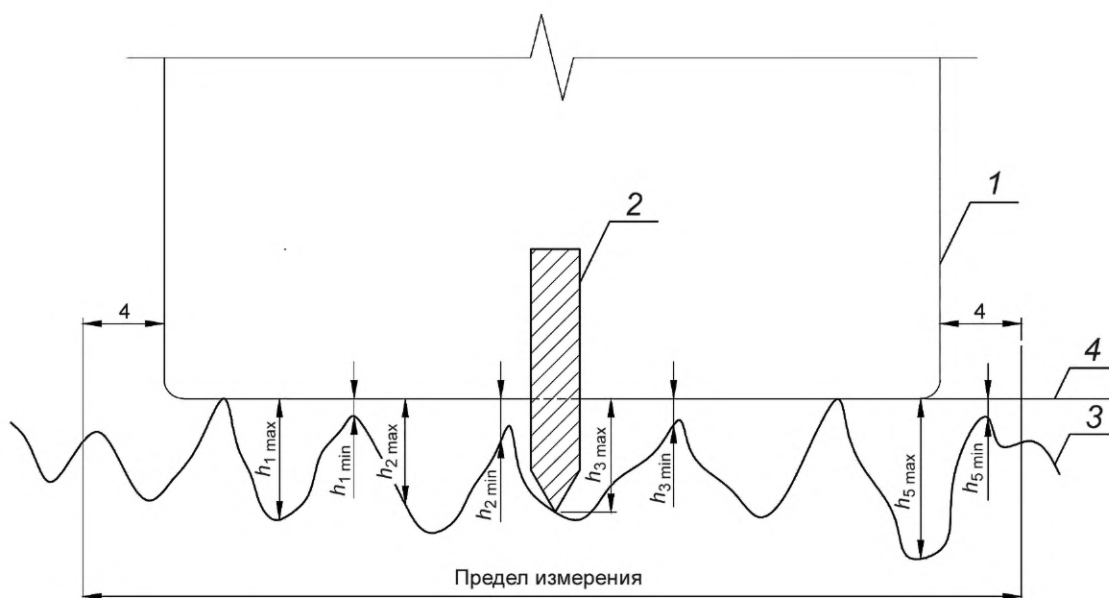
Рисунок 1 — Схема проведения измерений на профиле поверхности
