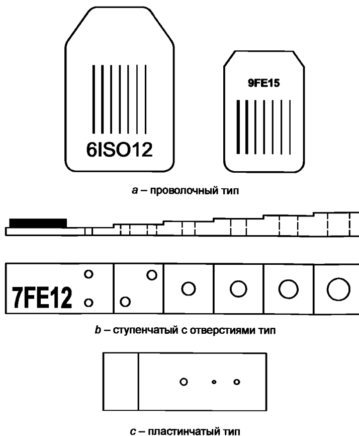
Рисунок 4 — Типы индикаторов качества изображения (IQI)
