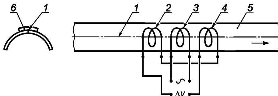
Рисунок 2 — Упрощенная схема вихретокового метода контроля с дисконной катушкой
