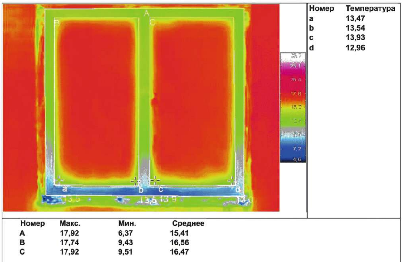
Рисунок А.8 — Распределение температурных полей на испытуемой конструкции
