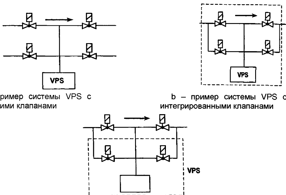
с — пример системы VPS с частично интегрированными клапанами
