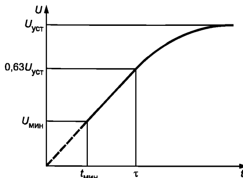
Рисунок 2 — Кривая натекания
