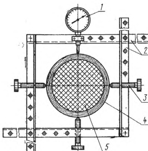
1 – индикатор; 2 – раздвижные планки; 3 – установочные винты; 4 – втулка; 5 – парафин
