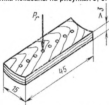
P_r – действие нагрузки в радиальном направлении
