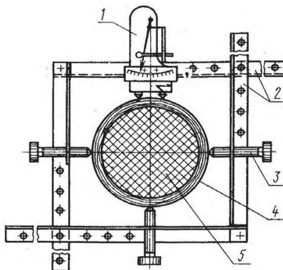
1 – тензометр; 2 – раздвижные планки; 3 – установочные винты; 4 – втулка; 5 – парафин
