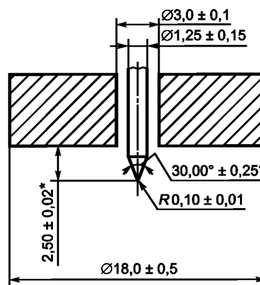
Рисунок 2 — Индентор для дюрометра типа D
