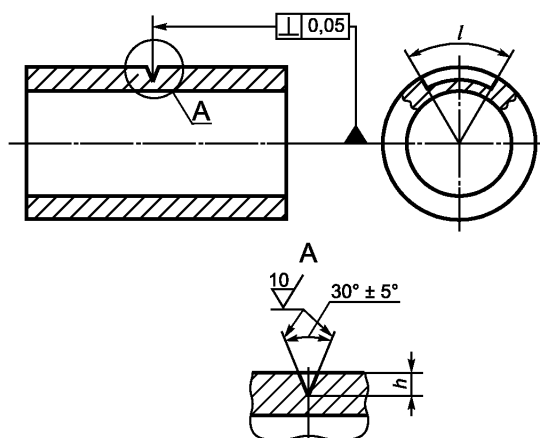
Рисунок 8 — Искусственный отражатель типа риски
