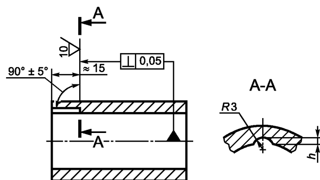
Рисунок 9 — Искусственный отражатель типа сегментного отражателя
