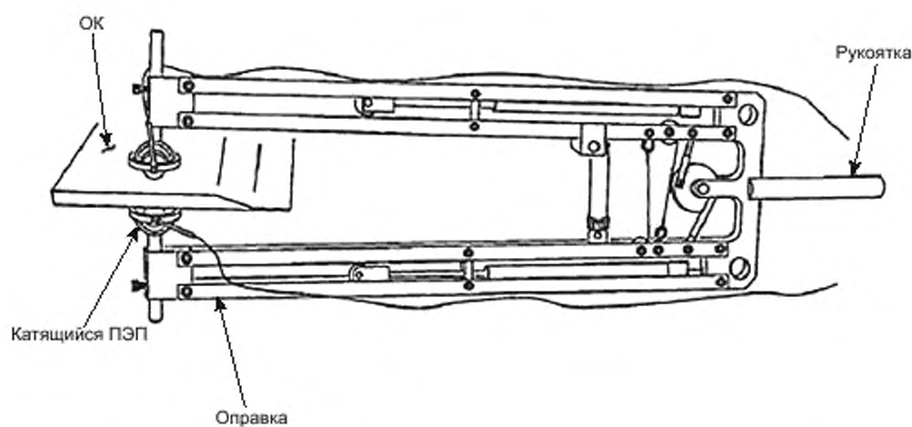
Рисунок 3 — Ручной теневой контроль с использованием катящихся преобразователей
