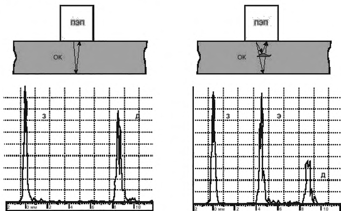
Рисунок 1 — Принцип выявления дефектов эхометодом
