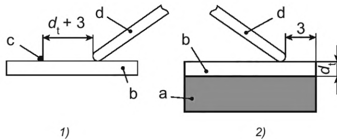
а — подложка; б — пластмассовый лист; с — провод; d — электрод
