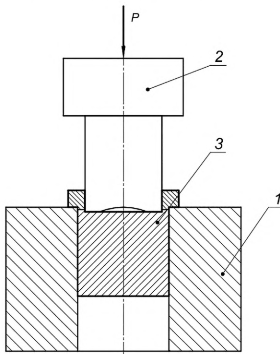
1 — матрица; 2 — пуансон; 3 — испытуемый образец
