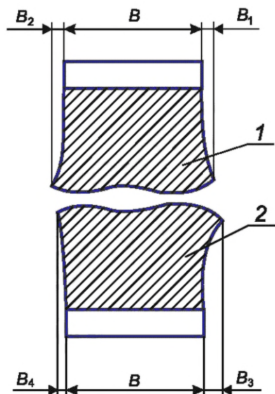
Рисунок 1 — Половины разрушенного в процессе испытания образца, соединенные для измерения бокового расширения
