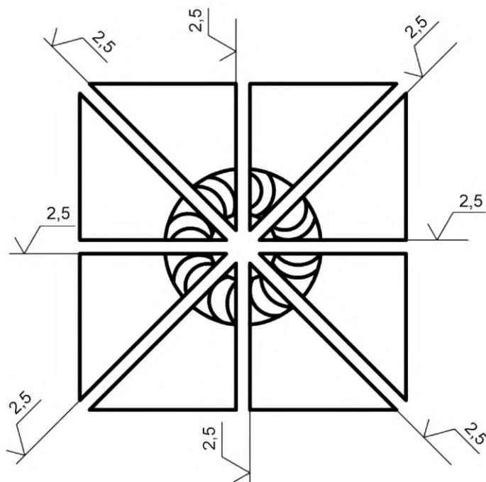
а) Вид сверху на пробу, разрезанную на макрошлифы
