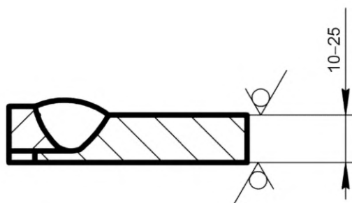
в) Рекомендуемые размеры макрошлифа
