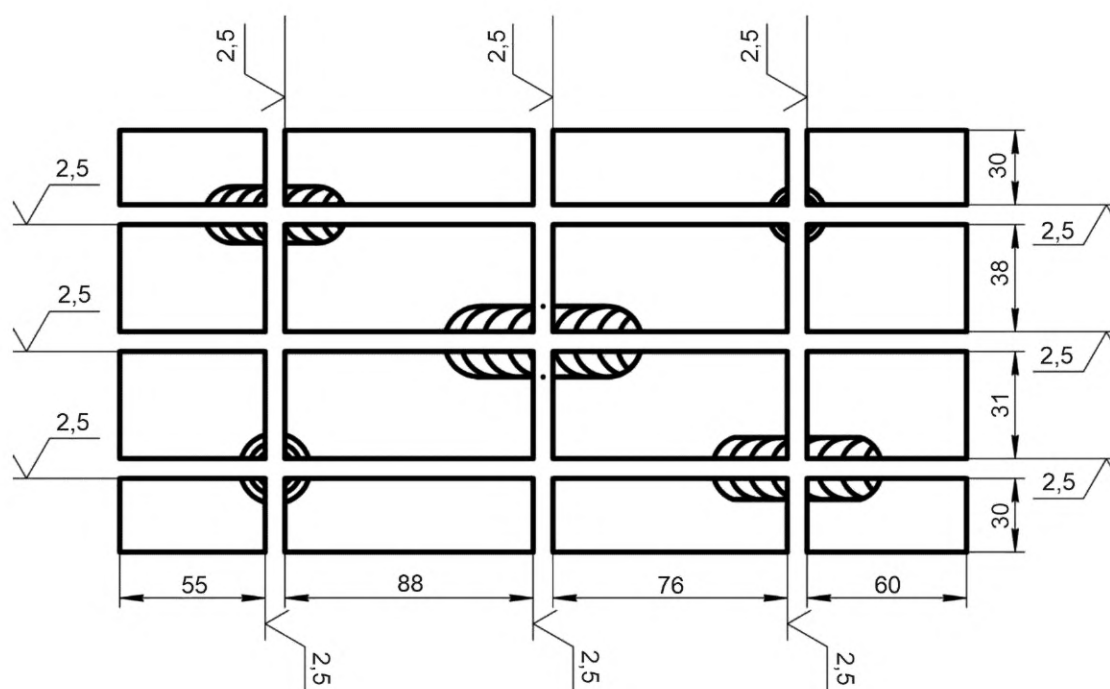
Рисунок 7 — Схема разрезки заваренной пробы
