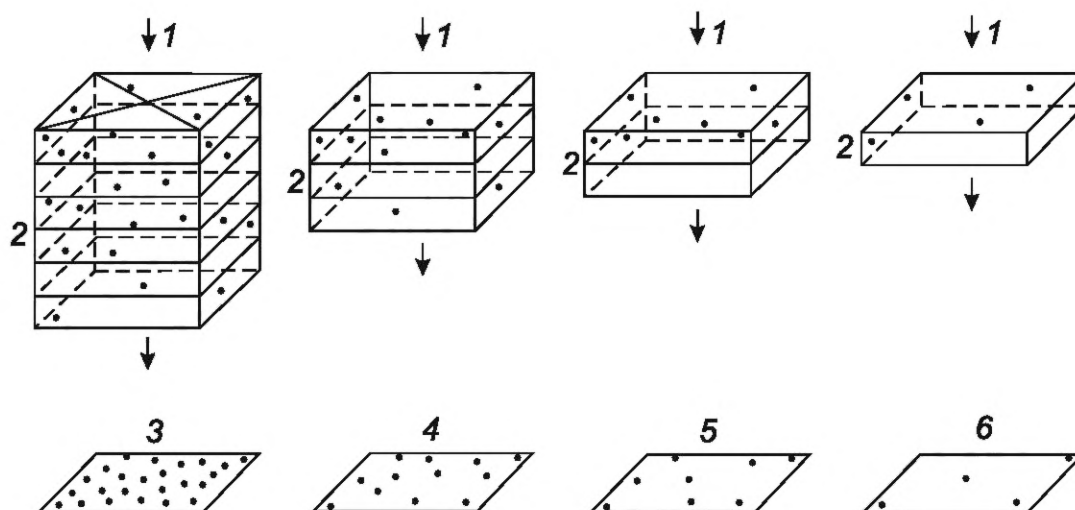
1 — направление рентгеновского излучения; 2 — четыре поры на единицу объема; 3 — шестислойная толщина; 4 — трехслойная толщина; 5 — двухслойная толщина; 6 — однослойная толщина
