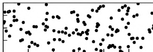
Рисунок А.8 — 8 % поверхности, 122 поры, d = 1 мм
