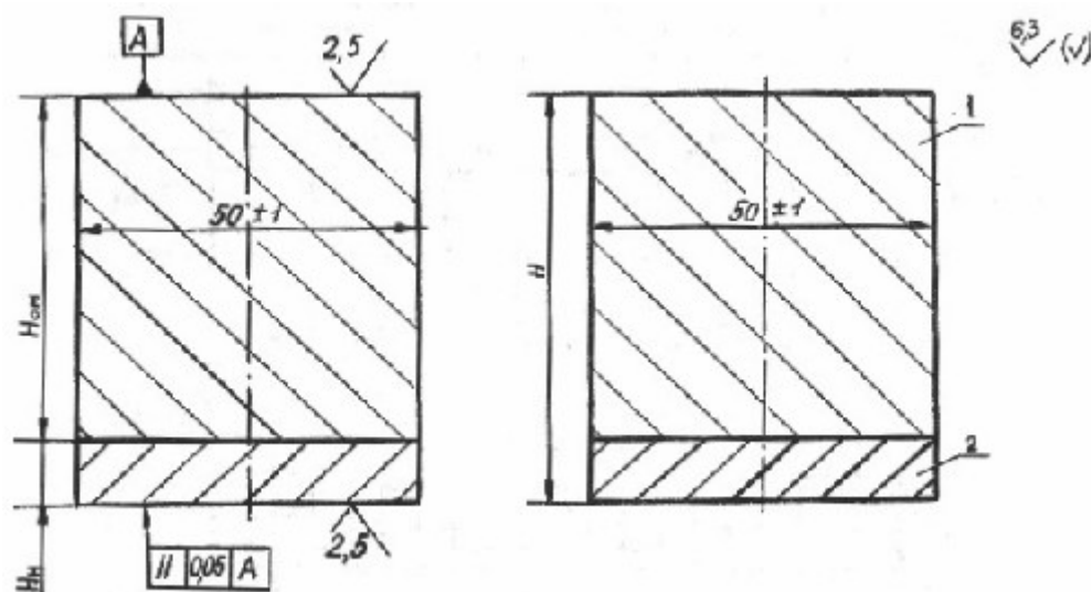
Рис.3. Стандартный образец предприятия тип ТБ1 для настройки прибора при измерении толщины биметалла: 1 - основной металл; 2 - антикоррозионное покрытие; H = (1 \pm 0,1) H_0 ; H_{ом} = (1 \pm 0,1) H_{ом0} ; H_n = H_{мин} + 2 мм, где H_0 , H_{ом0} - номинальные значения толщин биметалла и основного металла соответственно; H - минимальная толщина антикоррозионного покрытия
