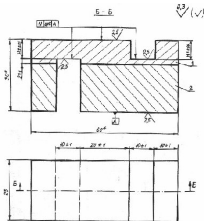
Рис.6. Стандартный образец предприятия тип ТНЗ для настройки дефектоскопа при измерении толщины антикоррозионного покрытия как со стороны основного металла, так и со стороны покрытия ( x - размер для справки): 1 - антикоррозионное покрытие; 2 - основной металл; H=H^{\pm 1} , где H_n - номинальная толщина антикоррозионного покрытия
