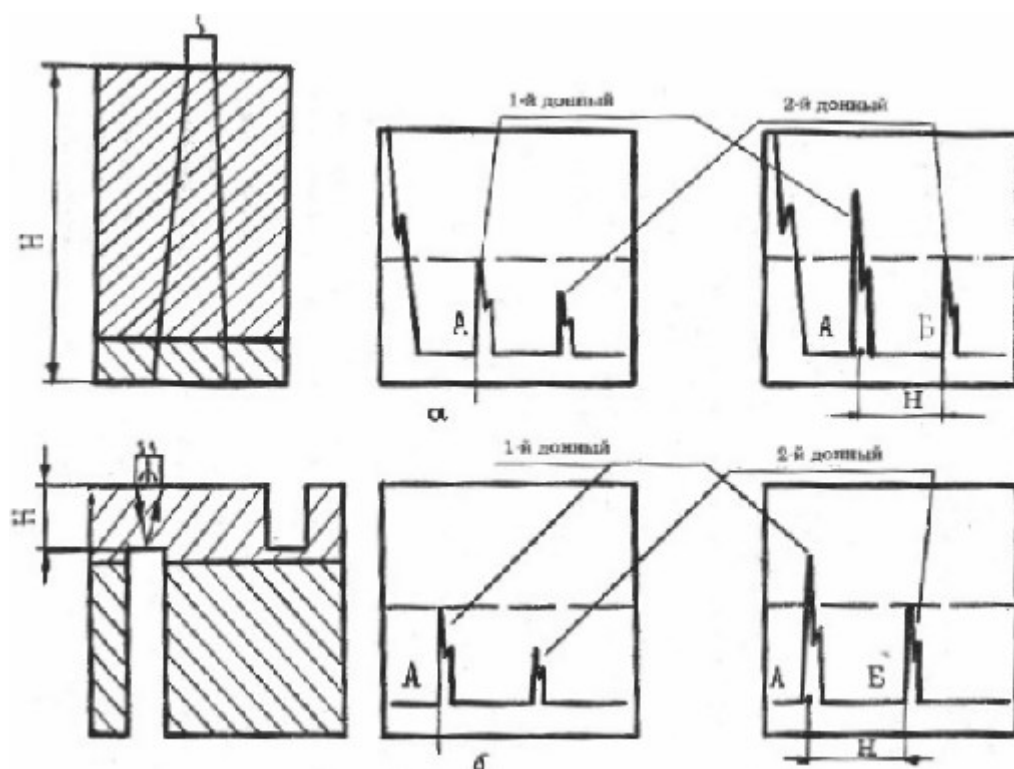
Рис.9. Схема настройки на скорость звука в изделии по образцам ТБ1 (а) и ТНЗ (б)
