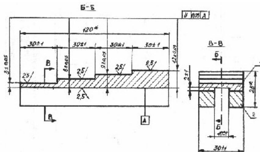
Рис. 5. Стандартный образец предприятия тип ТН2 для настройки дефектоскопа при измерении толщины антикоррозионного покрытия со стороны покрытия (х - размер для справки): 1 - антикоррозионное покрытие; 2 - основной металл
