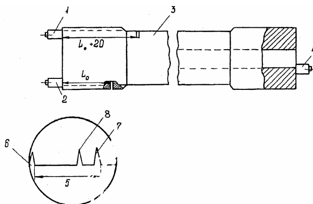
Рис. 3. Схема настройки скорости развертки и чувствительности дефектоскопа при контроле резьбовых участков шпильки:
