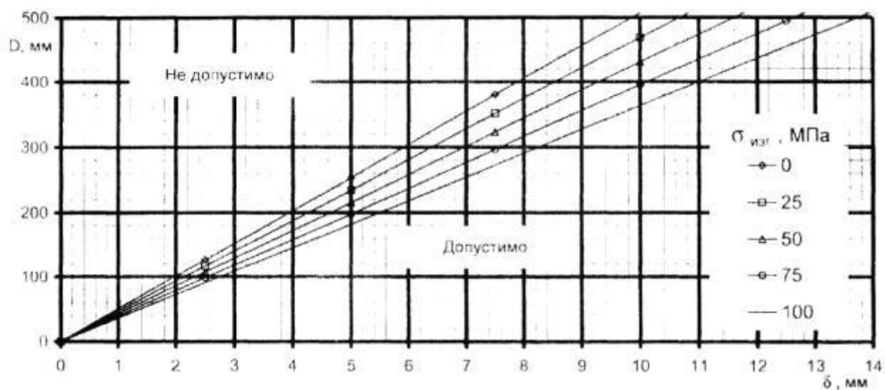
Рис. 7. Зависимость толщины стенки трубопровода от диаметра при различных значениях напряжения изгиба с запасом прочности n = 2,5
