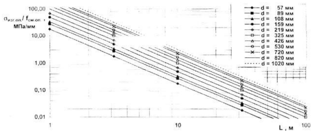
Рис. 4. Зависимость напряжения изгиба при консольном закреплении трубопровода:
