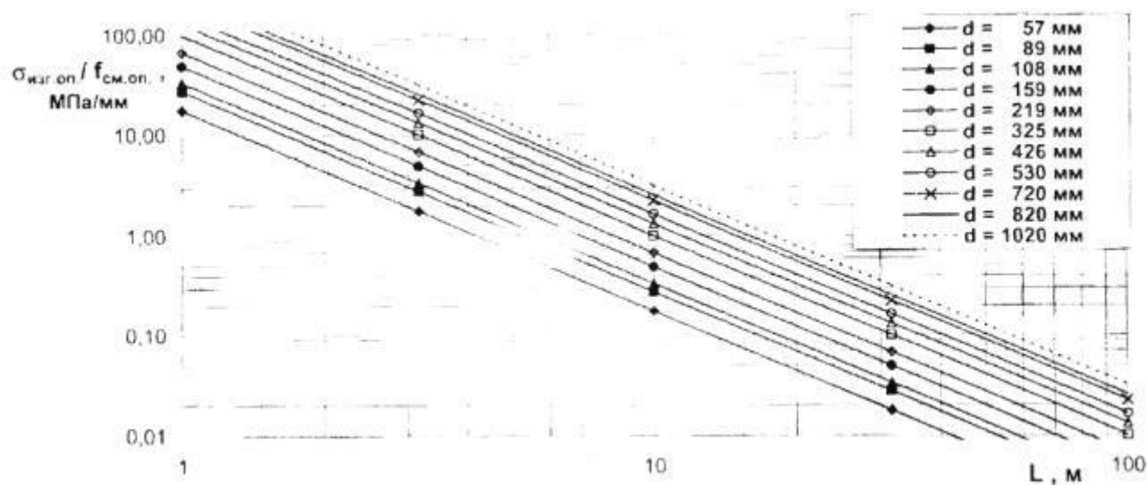
Рис. 3. Зависимость напряжения изгиба от смещения опор для шарнирно опертого трубопровода:
