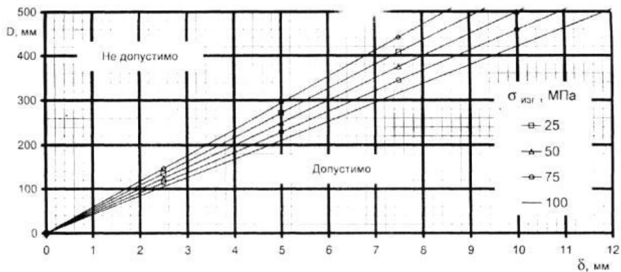
Рис. 6. Зависимость толщины стенки трубопровода от диаметра при различных значениях напряжения изгиба с запасом прочности n = 2,5
