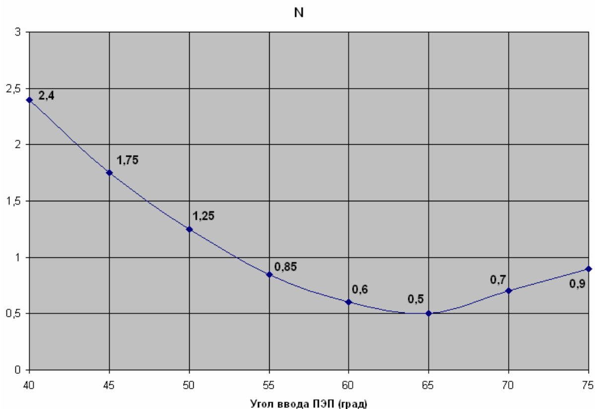
Рис.3. Зависимость коэффициента N от угла ввода ультразвукового наклонного преобразователя.
